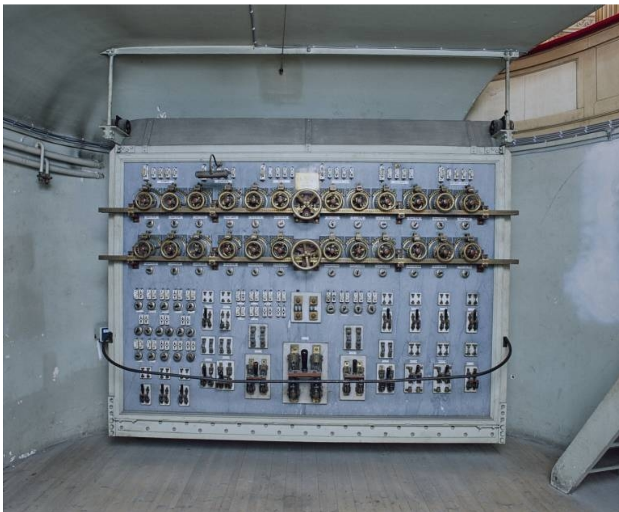
Sous-sol : tableau de commande (jeu d'orgue), en 1996.
