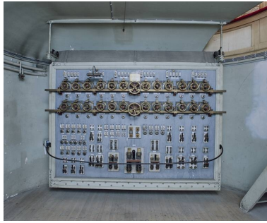
Sous-sol : tableau de commande (jeu d'orgue), en 1996. Phot. Michel Rosso IVR26_19967100714XA
