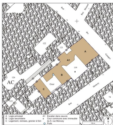
Plan masse et de situation. Extrait du plan cadastral, 1974, section AC. Dess. André Céréza IVR43_20102500050NUDA
