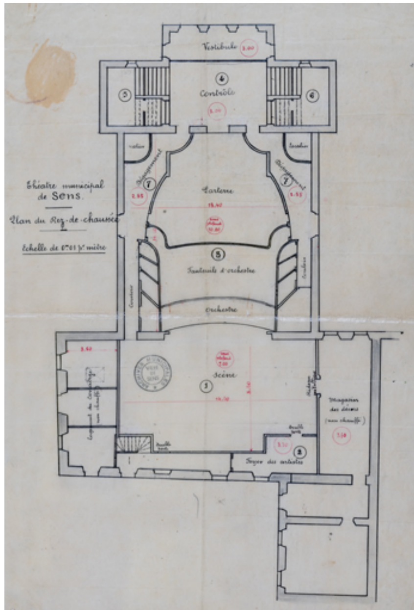
Théâtre municipal de Sens. Plan du rez-de-chaussée. S.d. [4e quart 19e siècle ?].
