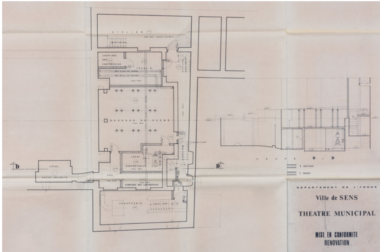
Théâtre municipal. Mise en conformité. Rénovation. APD. SC 1. Atelier, chaufferie, local accus-sécurité, local surpresseur, 2ème dessous de scène [détail]. 1978.
