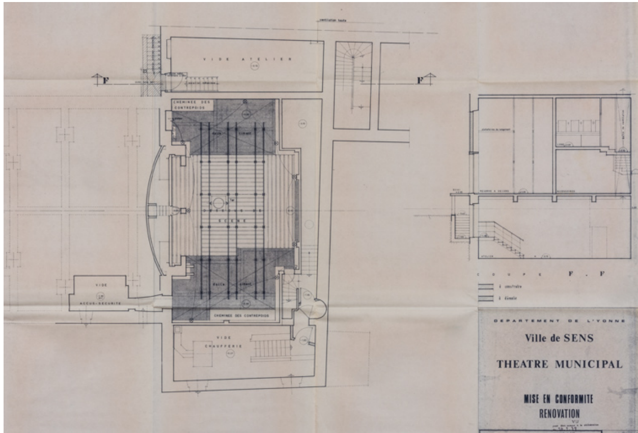
Théâtre municipal. Mise en conformité. Rénovation. APD. SC 2. Vide atelier, vide local accus, vide local chaufferie, 1er dessous de scène [détail]. 1978.
