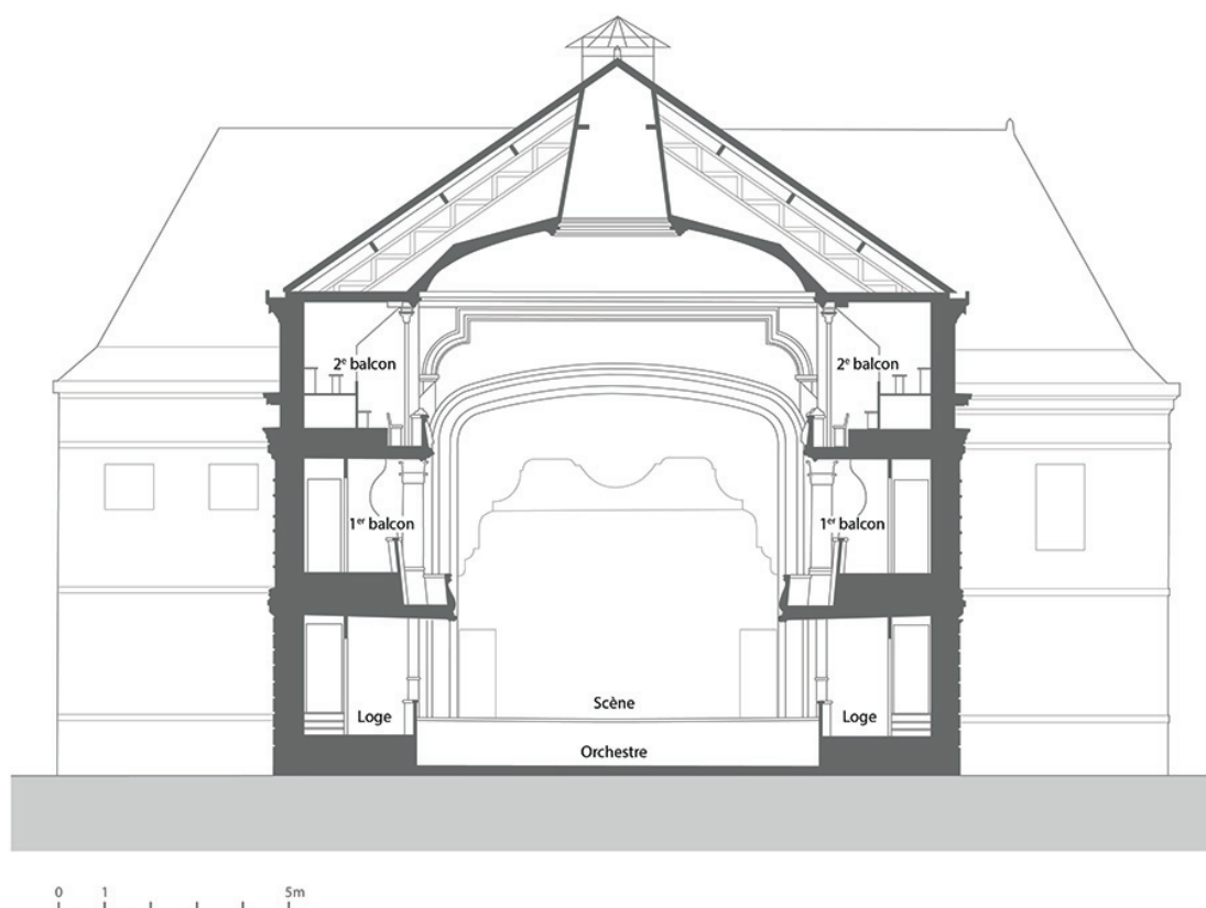
Coupe transversale. D'après le scan d'un dessin de C. Demangeat, vers 1978, fourni par le service Ingénierie et des Projets structurants de la ville de Sens.
