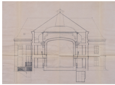
Théâtre municipal. Mise en conformité. Rénovation. APD. SC 8A. Coupes transversales sur salle et sur scène [détail : coupe sur la salle]. 1978. Phot. Pierre-Marie Barbe-Richaud, Autr. Camille Demangeat IVR26_20238900251NUC4A
