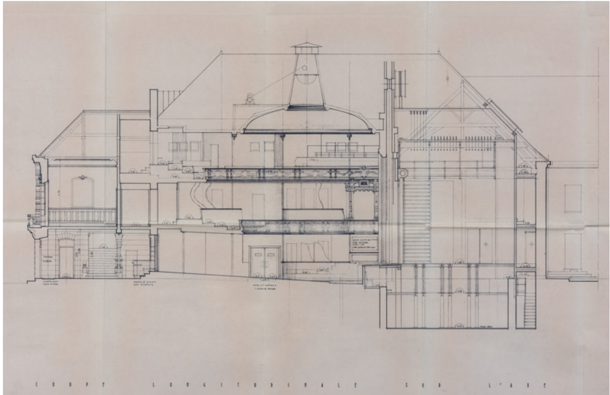
Théâtre municipal. Mise en conformité. Rénovation. APD. SC 7. Coupe longitudinale sur l'axe. 1978.
