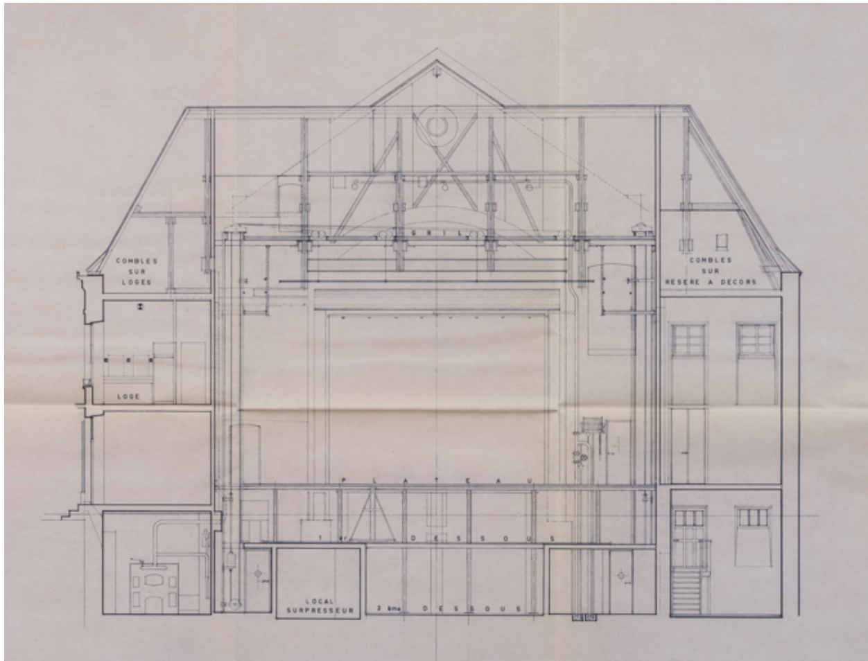
Théâtre municipal. Mise en conformité. Rénovation. APD. SC 8A. Coupes transversales sur salle et sur scène [détail : coupe sur la scène]. 1978.
