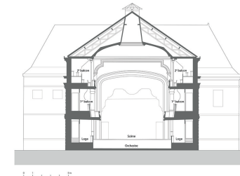
Coupe transversale. D'après le scan d'un dessin de C. Demangeat, vers 1978, fourni par
