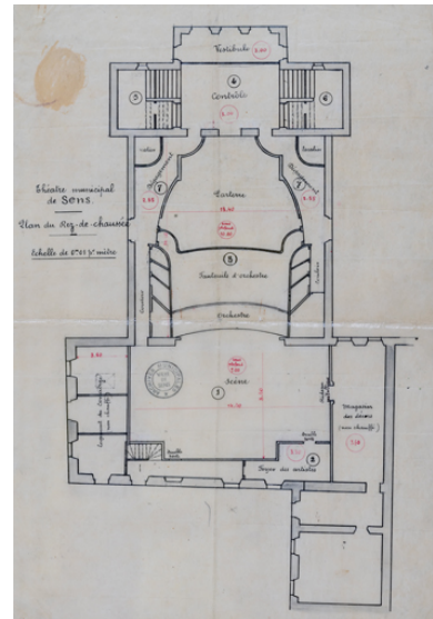
Théâtre municipal de Sens. Plan du rez-de-chaussée. S.d. [4e quart 19e siècle ?]. Phot. Pierre-Marie Barbe- Richaud, Autr. auteur inconnu IVR26_20238900245NUC4A
