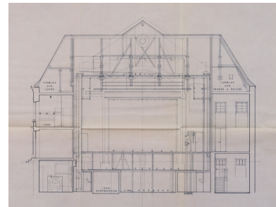
Théâtre municipal. Mise en conformité. Rénovation. APD. SC 8A. Coupes transversales sur salle et sur scène [détail : coupe sur la scène]. 1978. Phot. Pierre-Marie Barbe-Richaud, Autr. Camille Demangeat IVR26_20238900252NUC4A
