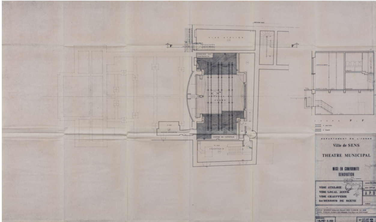
Théâtre municipal. Mise en conformité. Rénovation. APD. SC 2. Vide atelier, vide local accus, vide local chaufferie, 1er dessous de scène. 1978.
