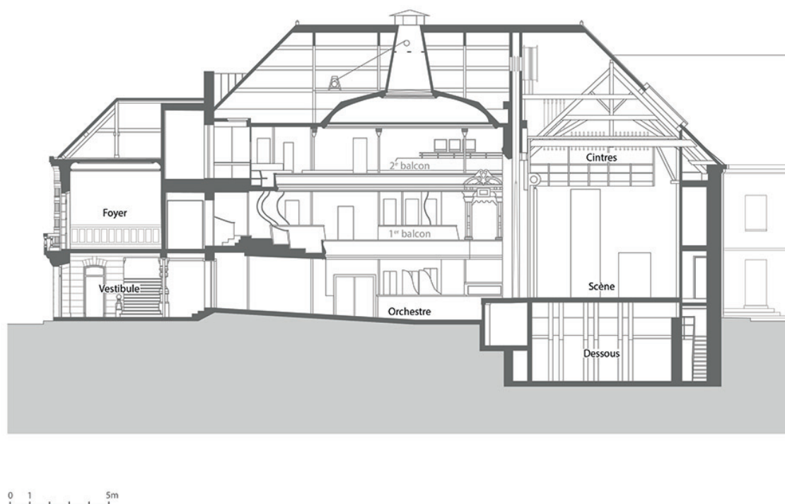
Coupe longitudinale. D'après le scan d'un dessin de C. Demangeat en 1978, fourni par le service Ingénierie et des Projets structurants de la ville de Sens.
