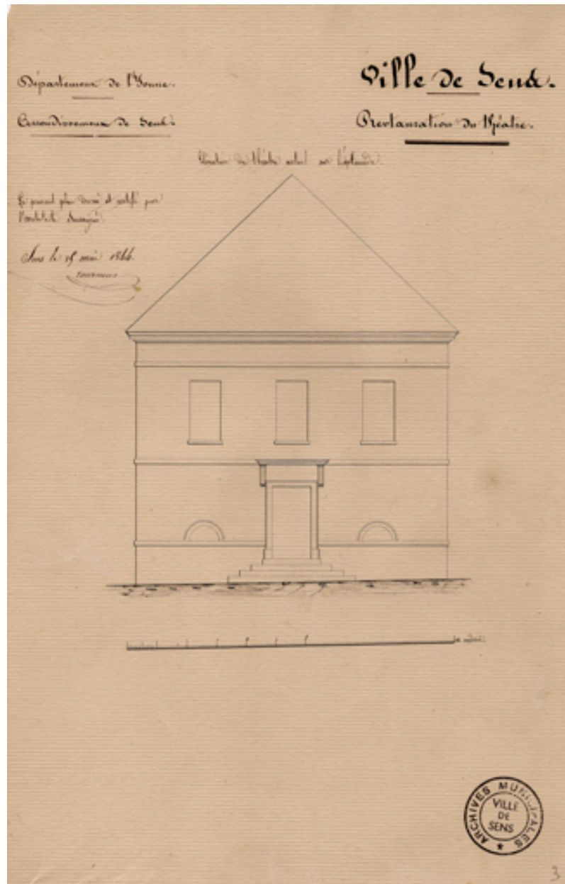
Restauration du théâtre. Elévation du théâtre actuel sur l'esplanade. 1844.
