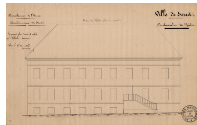
Restauration du théâtre. Elévation du théâtre au couchant. 1844. Phot. Pierre-Marie Barbe-Richaud, Autr. Jacques Athanase Tourneur IVR26_20238900277NUC4A
