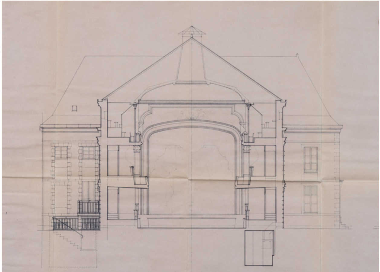
Théâtre municipal. Mise en conformité. Rénovation. APD. SC 8A. Coupes transversales sur salle et sur scène [détail : coupe sur la salle]. 1978.
