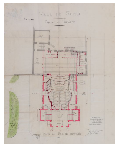
Projet de théâtre. Plan du rez-de-chaussée. 1879. Phot. Pierre-Marie Barbe- Richaud, Autr. Horace Lefort IVR26_20238900240NUC2A
