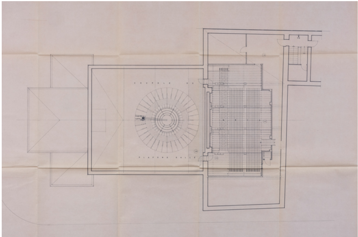
Théâtre municipal. Mise en conformité. Rénovation. APD. SC 6A. Coupole salle niveau gril. 1978.
