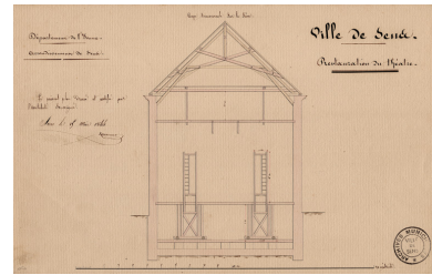
Restauration du théâtre. Coupe transversale sur la scène [projet]. 1844. Phot. Pierre-Marie Barbe-Richaud, Autr. Jacques Athanase Tourneur IVR26_20238900284NUC4A
