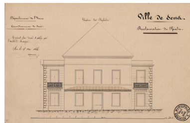
Restauration du théâtre. Elévation sur l'esplanade [projet]. 1844. Phot. Pierre-Marie Barbe-Richaud, Autr. Jacques Athanase Tourneur IVR26_20238900280NUC4A
