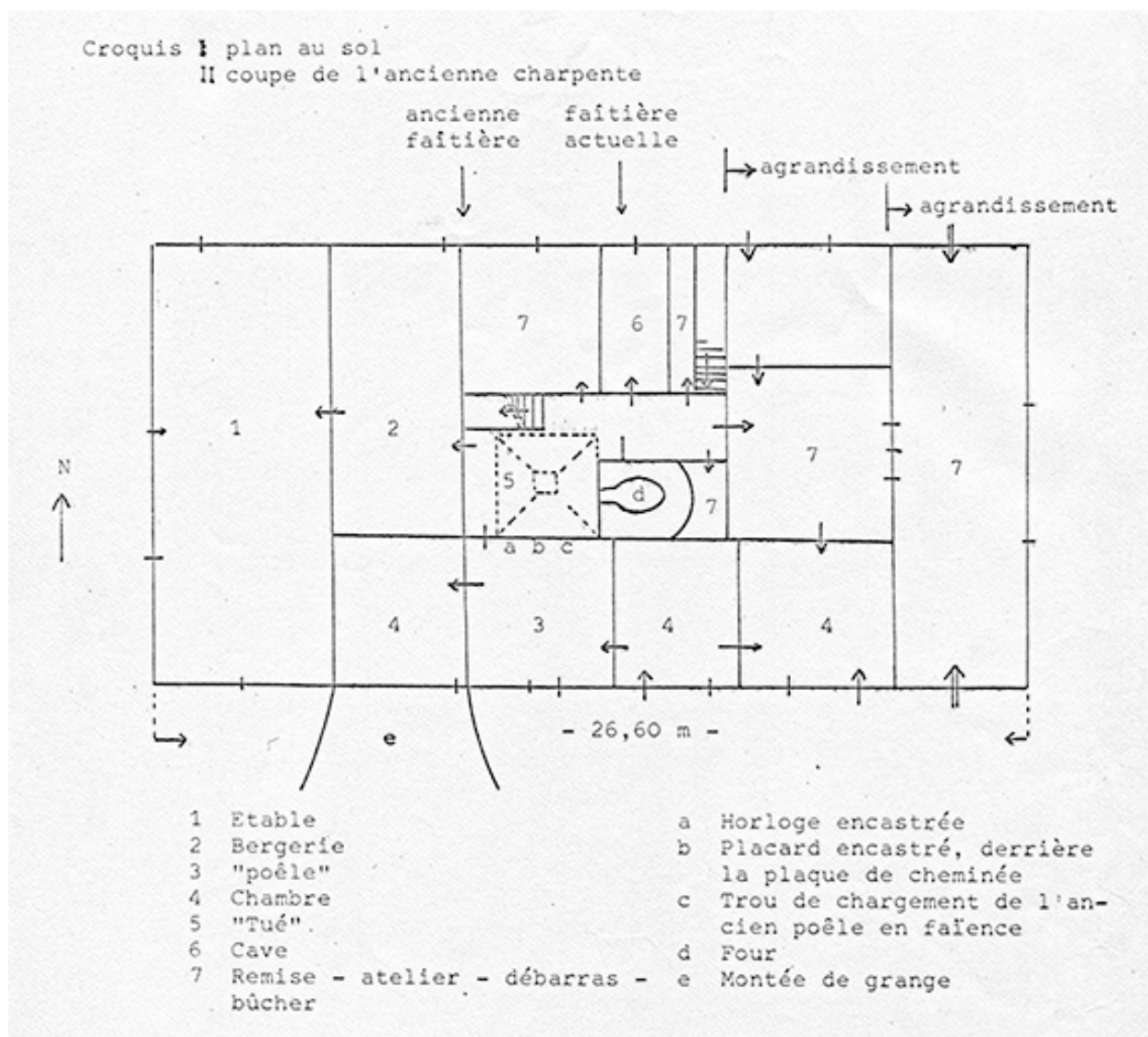
Croquis : plan au sol, 23 août 1976.
