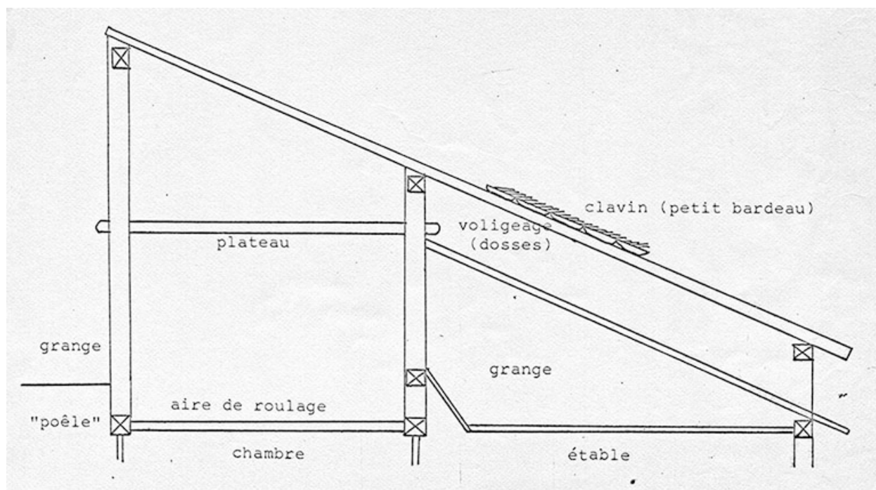
Croquis : coupe de l'ancienne charpente, 23 août 1976.
