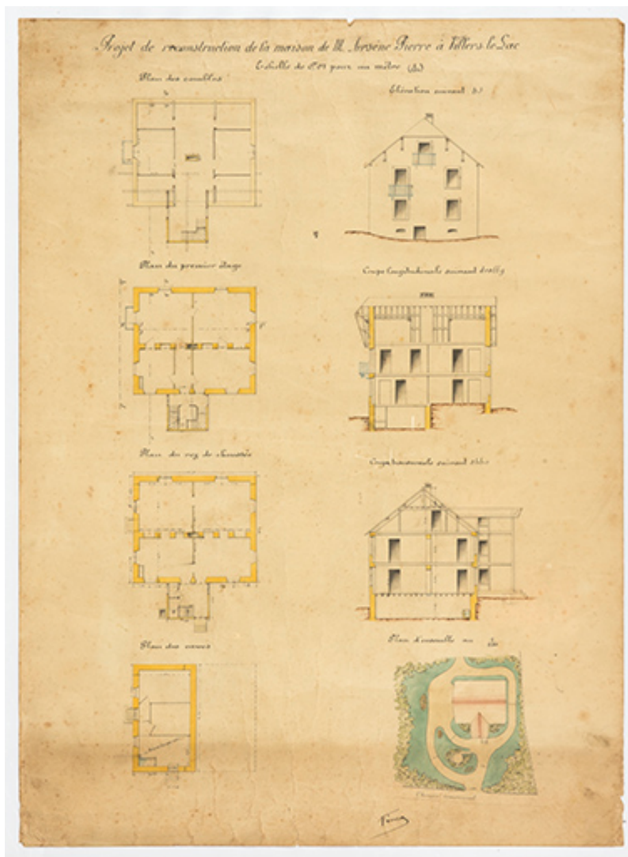
Projet de reconstruction de la maison de M. Arsène Pierre à Villers-le-Lac, 1er quart 20e siècle.
