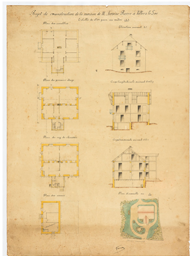
Projet de reconstruction de la maison de M. Arsène Pierre à Villers-le-Lac, 1er quart 20e siècle. Phot. Sonia Dourlot, Autr. Viney IVR43_20162501737NUC4A
