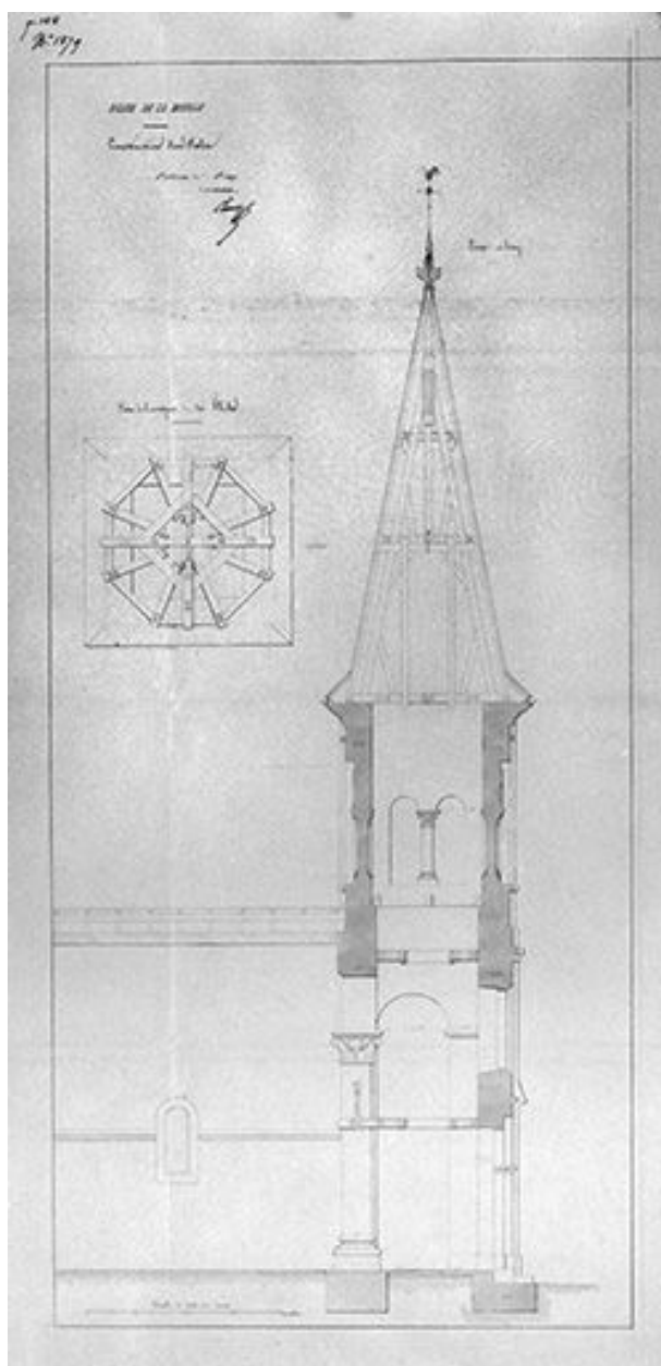
Construction d'un clocher : coupe longitudinale, 1849.
