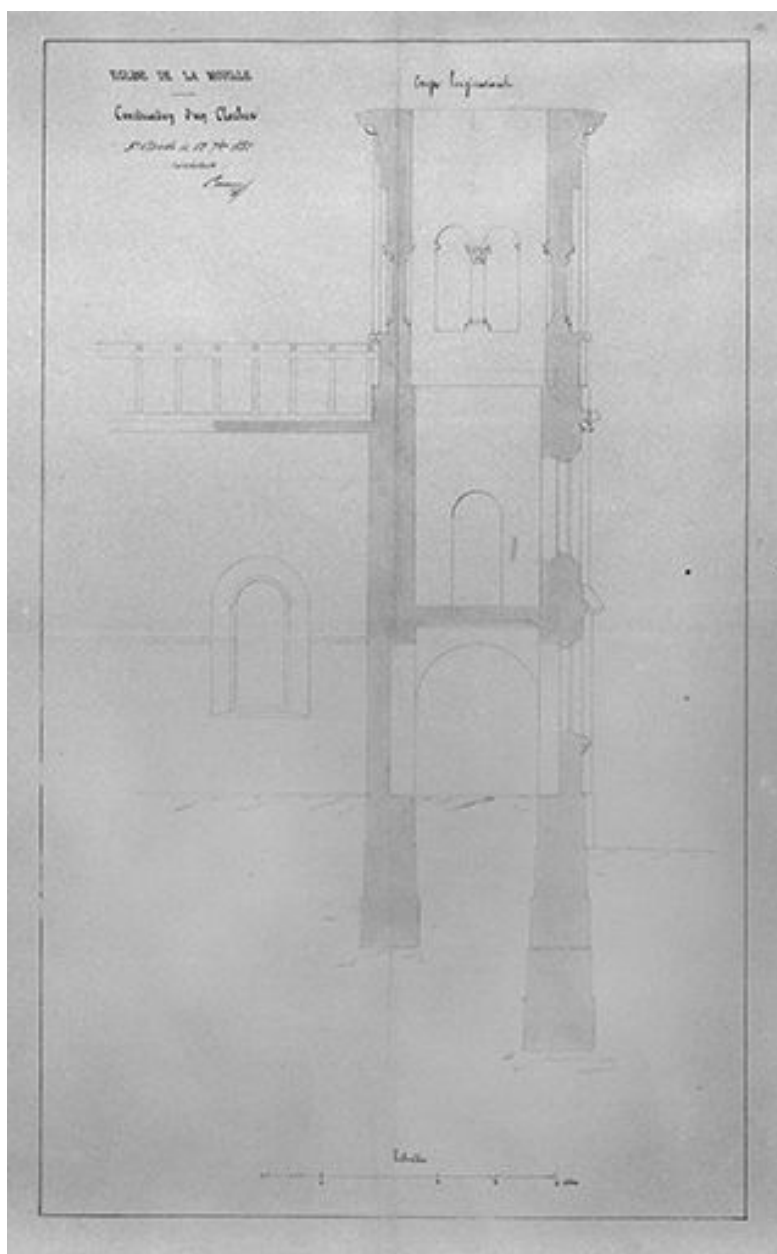
Construction d'un clocher : coupe longitudinale, 1850.
