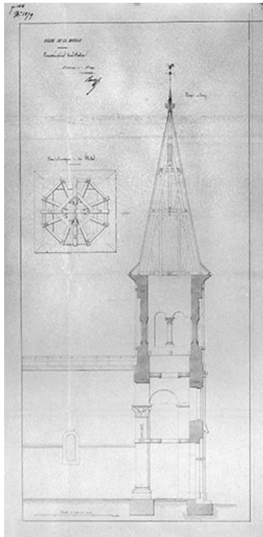
Construction d'un clocher : coupe longitudinale, 1849. Phot. Jérôme Mongreville, Phot. Auguste Comoy IVR43_20013900321V
