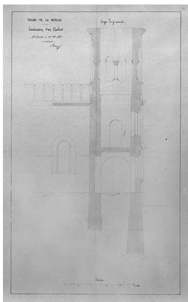
Construction d'un clocher : coupe longitudinale, 1850. Phot. Jérôme Mongreville, Phot. Auguste Comoy IVR43_20013900323V
