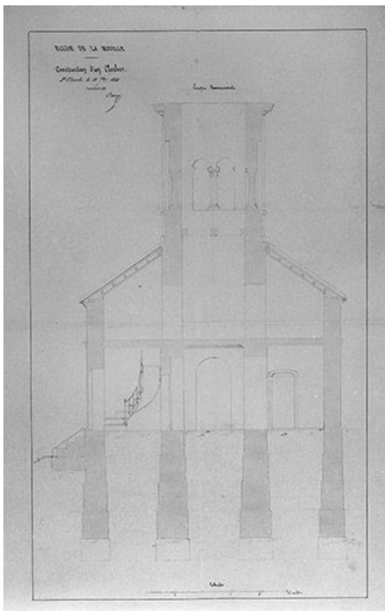
Construction d'un clocher : coupe transversale, 1850.
