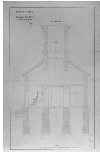
Construction d'un clocher : coupe transversale, 1850. Phot. Jérôme Mongreville, Phot. Auguste Comoy IVR43_20013900327V
