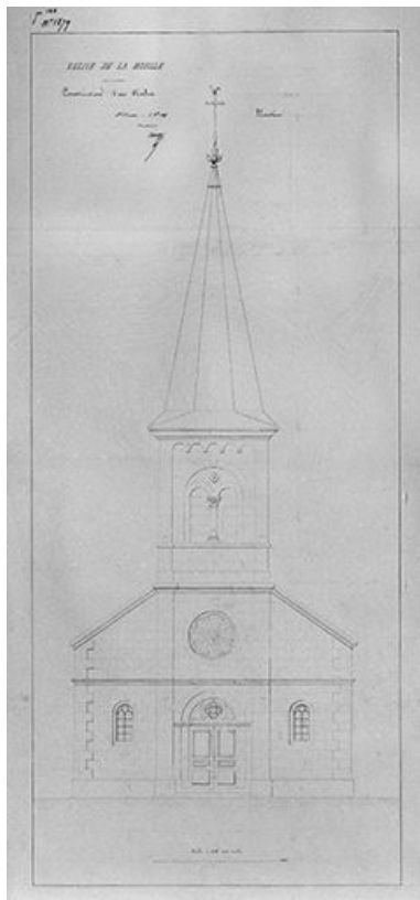
Construction d'un clocher : élévation, 1849. Phot. Jérôme Mongreville, Phot. Auguste Comoy IVR43_20013900334V
