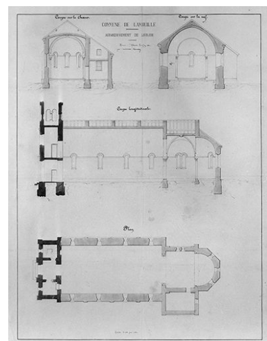
Agrandissement de l'église : plan, coupes longitudinales, sur le chœur et sur la nef, 1864. Phot. Jérôme Mongreville, Phot. Auguste Comoy IVR43_20013900336V
