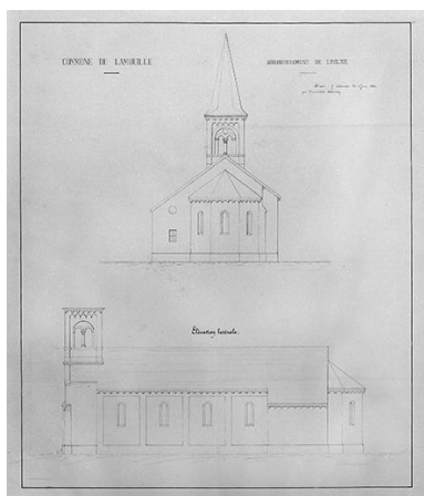
Agrandissement de l'église : plan, coupes longitudinales, sur le chœur et sur la nef, 1864. Phot. Jérôme Mongreville, Phot. Auguste Comoy IVR43_20013900335V
