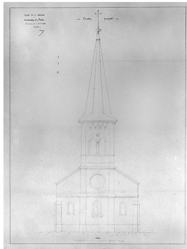
Construction d'un clocher : élévation principale, 1850. Phot. Jérôme Mongreville, Phot. Auguste Comoy IVR43_20013900322V
