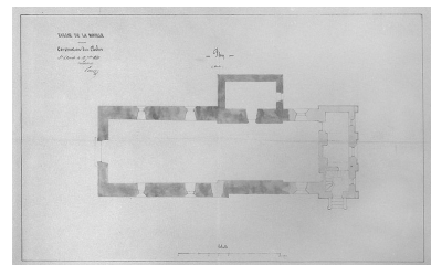
Construction d'un clocher : plan, 1850. Phot. Jérôme Mongreville, Phot. Auguste Comoy IVR43_20013900324V
