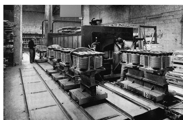
Faïencerie des Capucins, Salins-les-Bains : le four de cuisson des décors, [3e quart 20e siècle]. Phot. Jérôme Mongreville IVR43_19973900288X
