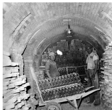
Briqueterie et tuilerie Emile Jacob, Commenailles : déchargement du four Hoffmann, 1955. Phot. Jérôme Mongreville IVR43_19893900065X
