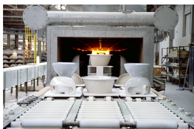
Usine de porcelaine Idéal Standard, Dole : défournement en bout du four tunnel. Phot. Laurent Poupard IVR43_19893901141ZA
