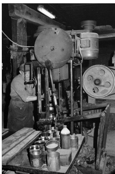
Poterie et briqueterie Martin, Etrepigny : mouleuse à pots de fleur Crochon. Phot. Laurent Poupard IVR43_19883900354Z
