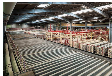
Tuilerie et briqueterie Migeon, à Lantenne-Vertière : unité de fabrication UL 2. La partie supérieure du four piscine occupe le premier plan. Phot. Jérôme Mongreville IVR43_20152501332NUC4A
