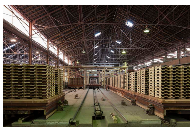
Tuilerie et briqueterie Migeon, à Lantenne-Vertière : unité de fabrication UL 1. Chariots de four. Phot. Jérôme Mongreville IVR43_20152501349NUC4A
