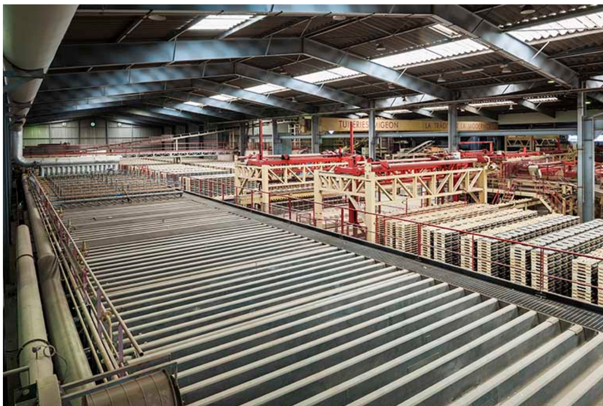
Tuilerie et briqueterie Migeon, à Lantenne-Vertière : unité de fabrication UL 2. La partie supérieure du four piscine occupe le premier plan.
