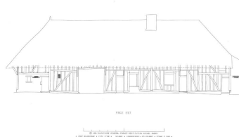
façade est
