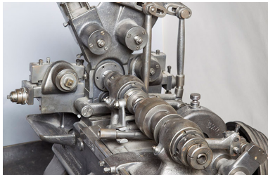
Poupée mobile et arrière de la lunette. Phot. Jérôme Mongreville IVR43_20142500731NUC2A
