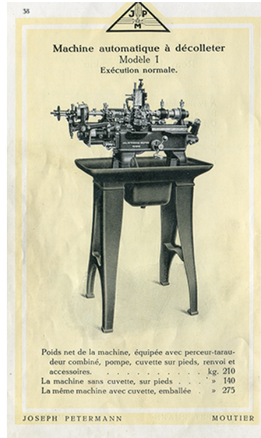
Machine automatique à décolleter modèle 1, exécution normale, années 1920. IVR43_20142500912NUC2A
