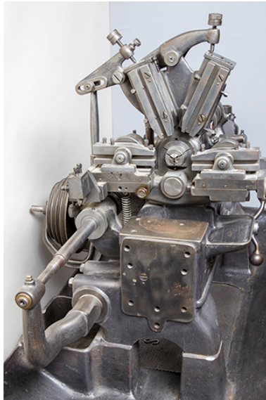
Espace d'usinage (vue d'ensemble plongeante). Phot. Jérôme Mongreville IVR43_20142500728NUC2A
