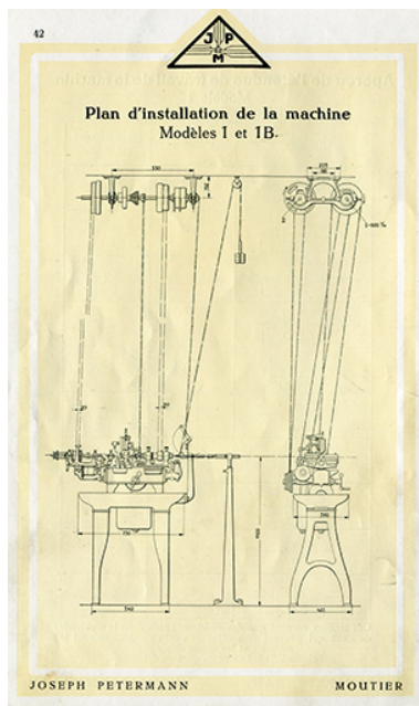
Plan d'installation de la machine modèles 1 et 1B, années 1920. IVR43_20142500914NUC2A
