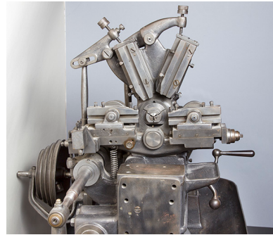
Espace d'usinage : lunette sur bascule avec ses quatre porte-burins. Phot. Jérôme Mongreville IVR43_20142500729NUC2A
