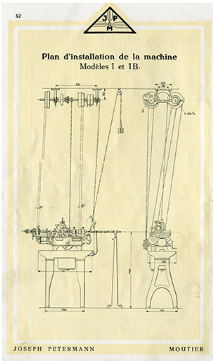
Plan d'installation de la machine modèles 1 et 1B, années 1920.
