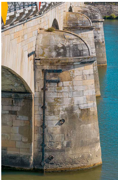
Détail des arrière-becs du pont et de l'échelle de crue. Phot. Thierry Kuntz IVR26_20217100568NUC2A
