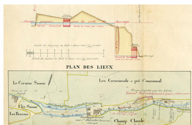
Plan et nivellement relatifs à la demande en changement de destination d'une usine par le sieur Vermot Des Roches, propriétaire habitant de la commune de Montlebon, 1822.
