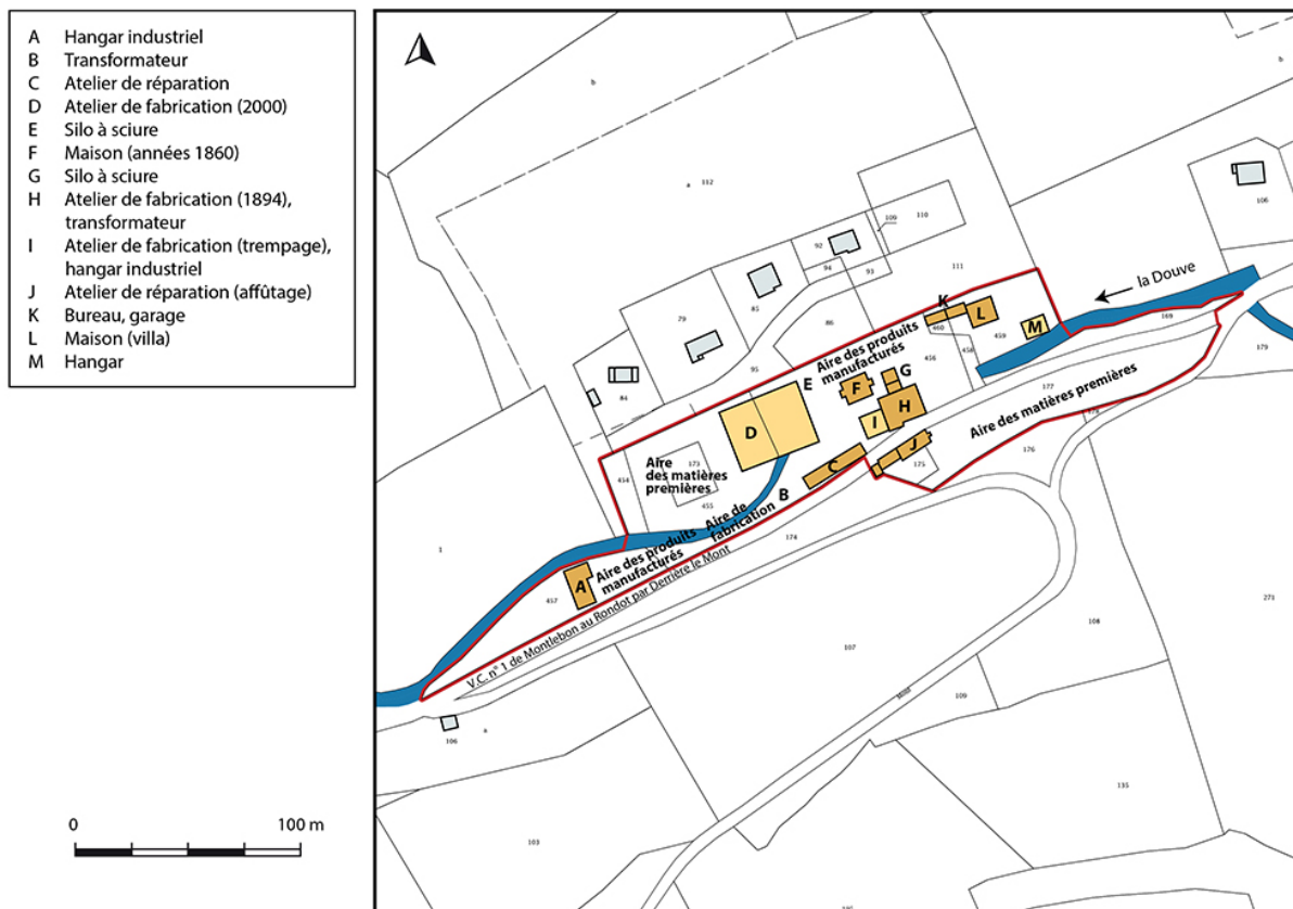
Plan-masse et de situation. Extrait du plan cadastral, 2017, section D, 1/2 500 agrandi à 1/2 000.
