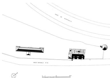
Plan-masse et de toiture. Dess. Alain Morelière IVR26_20125800028A3YY
