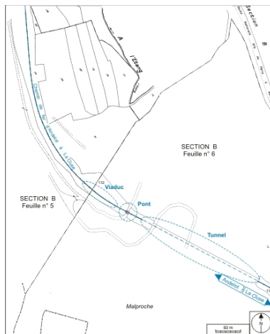
Plan-masse et de situation. Montage d'extraits du plan cadastral, 1985, section B, 5e et 6e feuilles, échelle 1:1250 réduite à 1:3000. Dess. André Céréza IVR43_20073900211NUDA
