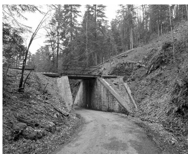
Pont, depuis la route côté rocher. Phot. Yves Sancey IVR43_20053900155X
