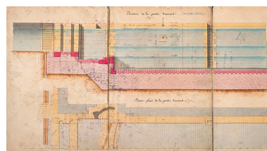
Construction de la dérivation de Port-sur-Saône - Ecluse à sas (1876) : élévation de la partie amont. Phot. Jérôme Mongreville, Autr. Gustave Bouvaist IVR43_20207000040NUC4A
