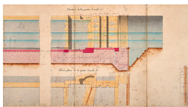
Construction de la dérivation de Port-sur-Saône - Ecluse à sas (1876) : élévation de la partie aval. Phot. Jérôme Mongreville, Autr. Gustave Bouvaist IVR43_20207000041NUC4A
