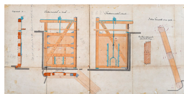
Construction de la dérivation de Port-sur-Saône - Portes d'Amont (1876). Phot. Jérôme Mongreville, Autr. Gustave Bouvaist IVR43_20207000054NUC4A
