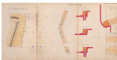
Construction de la dérivation de Port-sur-Saône - Ecluse à sas (1876) : tracé de l'appareil des buscs, scellement des faux- buscs et tracé des chardonnets. Phot. Jérôme Mongreville, Autr. Gustave Bouvaist IVR43_20207000048NUC4A
