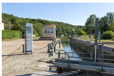
L'écluse et le poste de commande. Phot. Sonia Dourlot IVR43_20157000766NUC2A
