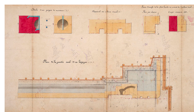
Construction de la dérivation de Port-sur-Saône - Ecluse à sas (1876) : détail d'une poignée de manoeuvre et plan de la partie aval d'un bajoyer. Phot. Jérôme Mongreville, Autr. Gustave Bouvaist IVR43_20207000043NUC4A
