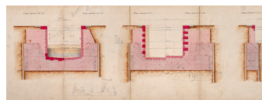
Construction de la dérivation de Port-sur-Saône - Ecluse à sas (1876) : vues en coupe (3). Phot. Jérôme Mongreville, Autr. Gustave Bouvaist IVR43_20207000046NUC4A
