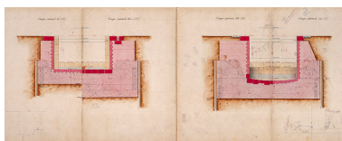
Construction de la dérivation de Port-sur-Saône - Ecluse à sas (1876) : vues en coupe (2). Phot. Jérôme Mongreville, Autr. Gustave Bouvaist IVR43_20207000045NUC4A
