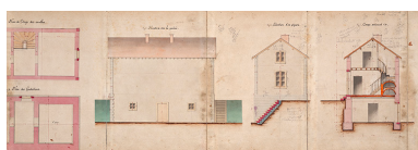
Construction de la dérivation de Port-sur-Saône - Maison éclusière (1876). Phot. Jérôme Mongreville, Autr. Gustave Bouvaist IVR43_20207000055NUC4A
