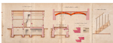
Construction de la dérivation de Port-sur-Saône - Maison éclusière (1876) Phot. Jérôme Mongreville, Autr. Gustave Bouvaist IVR43_20207000056NUC4A
