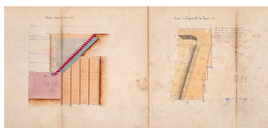
Construction de la dérivation de Port-sur-Saône - Ecluse à sas (1876) : vues en coupe (4). Phot. Jérôme Mongreville, Autr. Gustave Bouvaist IVR43_20207000047NUC4A
