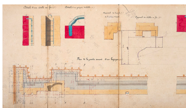
Construction de la dérivation de Port-sur-Saône - Ecluse à sas (1876) : détail d'une chelle en fer, détail d'une poignée d'échelle et plan de la partie amont d'un bajoyer. Phot. Jérôme Mongreville, Autr. Gustave Bouvaist IVR43_20207000042NUC4A
