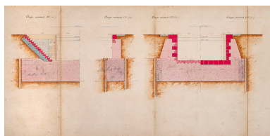
Construction de la dérivation de Port-sur-Saône - Ecluse à sas (1876) : vues en coupe (1). Phot. Jérôme Mongreville, Autr. Gustave Bouvaist IVR43_20207000044NUC4A
