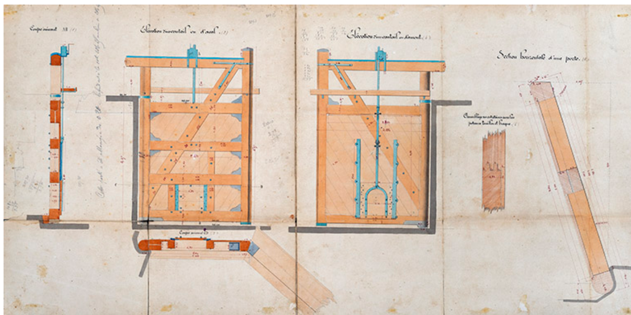
Construction de la dérivation de Port-sur-Saône - Portes d'Amont (1876).
