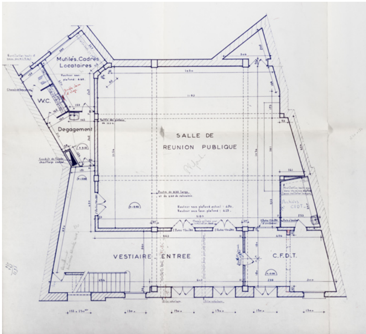
Bourse du Travail. Projet d'aménagement des salles. Rez de chaussée. 1969.
