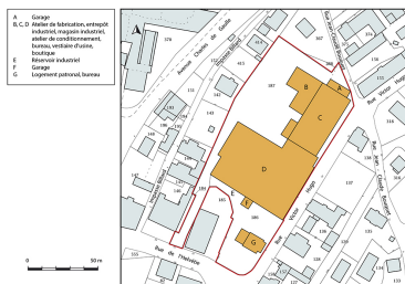
Plan-masse et de situation. Extrait du plan cadastral, 2018, section AF, 1/1 000. Dess. Bertrand Turina IVR43_20182501430NUDA
