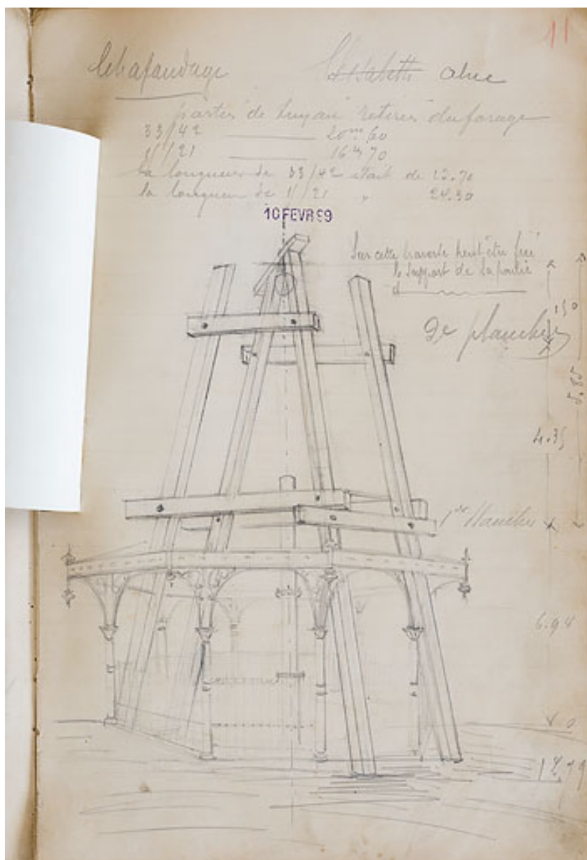
Échafaudage construit pour le forage de la source Alice en 1899.
