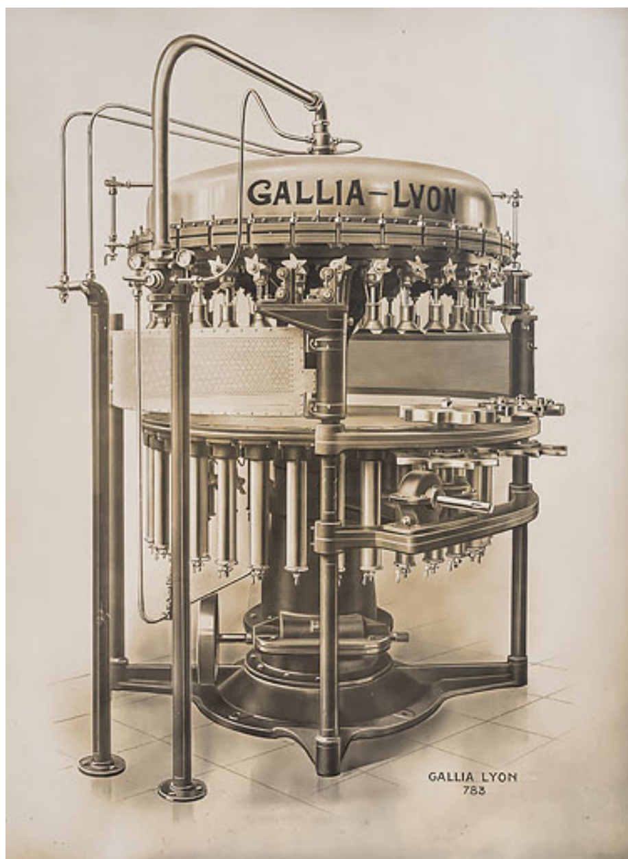
Modèle de machine d'embouteillage (Gallia-Lyon 783).
