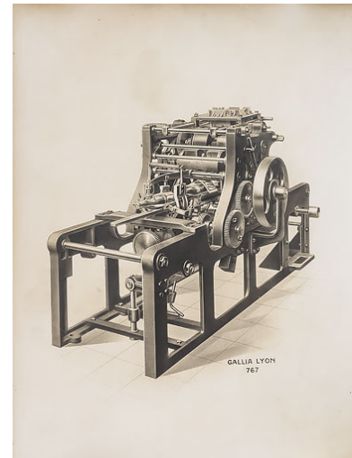
Modèle d'étiqueteuse (Gallia-Lyon 767). Autr. Gallia-Lyon, Phot. Pierre-Marie Barbe-Richaud IVR26_20205800222NUC2A
