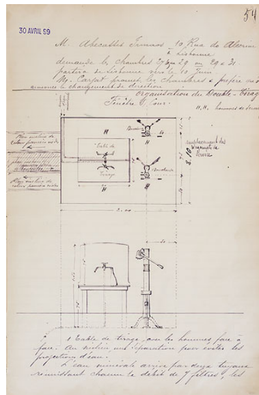
Schéma d'organisation du double- tirage à la fin du 19e siècle. Phot. Pierre-Marie Barbe- Richaud, Autr. Lucas IVR26_20205800227NUC2A
