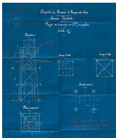
Plan et élévation du réservoir (1909).
