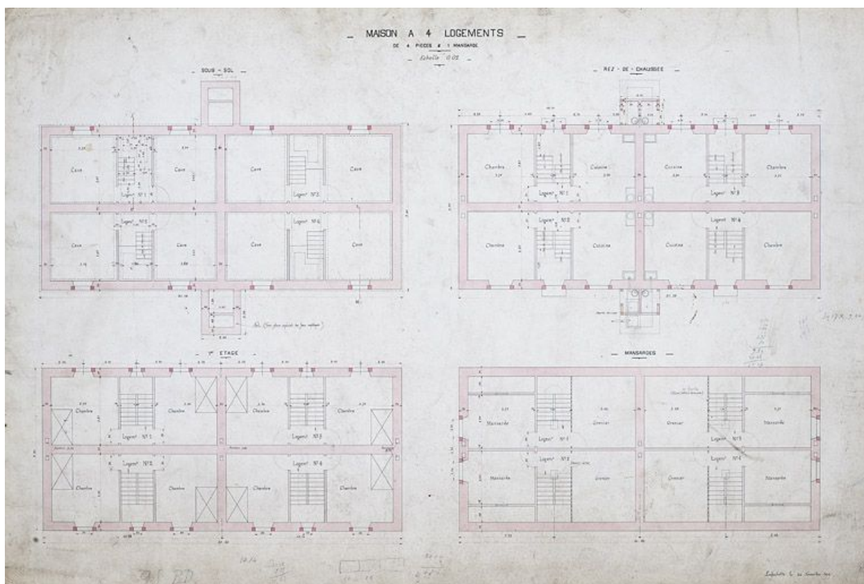
Maison à quatre logements de 4 pièces et une mansarde. Plan du sous-sol, du rez-de-chaussée, du 1er étage et des mansardes. Plan, encre, lavis, échelle 1/50, Lafeschotte, 26 novembre 1919.
