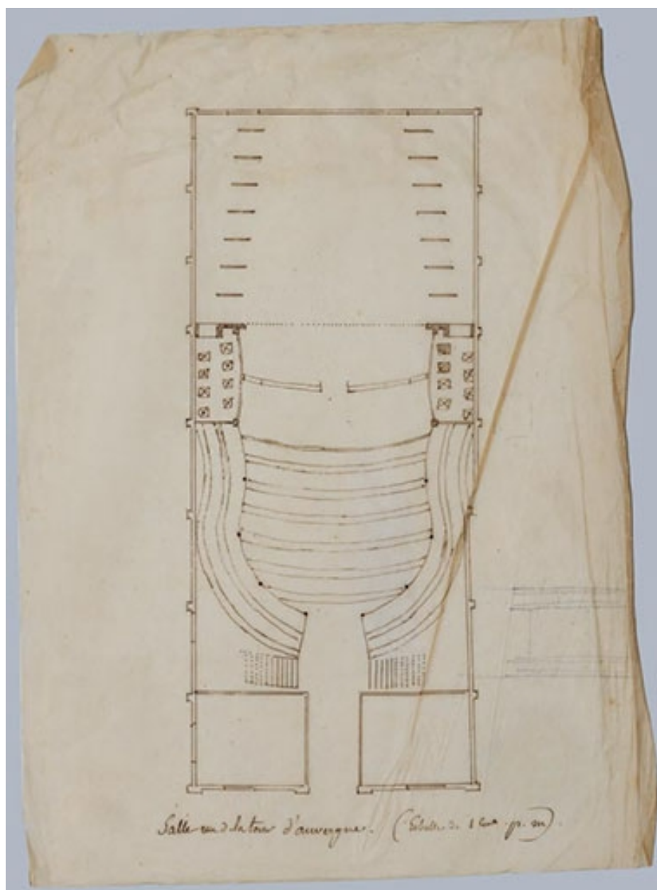
Salle rue de la tour d'auvergne. S.d. [1843 ?].
