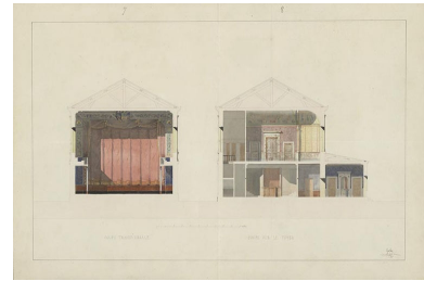
7. Coupe transversale [et] 8. Coupe sur le foyer. [Coupes et élévations par Grosley du théâtre projeté à Semur-en-Auxois]. S.d. [1843 ?]. Autr. Jean-Jacques Grosley IVR26_20222100281NUC2A
