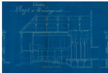
1721. Ville de Semur. Théâtre. Projet d'aménagement. [Détail :] Coupe longitudinale. S.d. [1903 ?]. Phot. Pierre-Marie Barbe-Richaud, Autr. Emile Wessbecher, Autr. Hector Marcorelles IVR26_20222100250NUC4A
