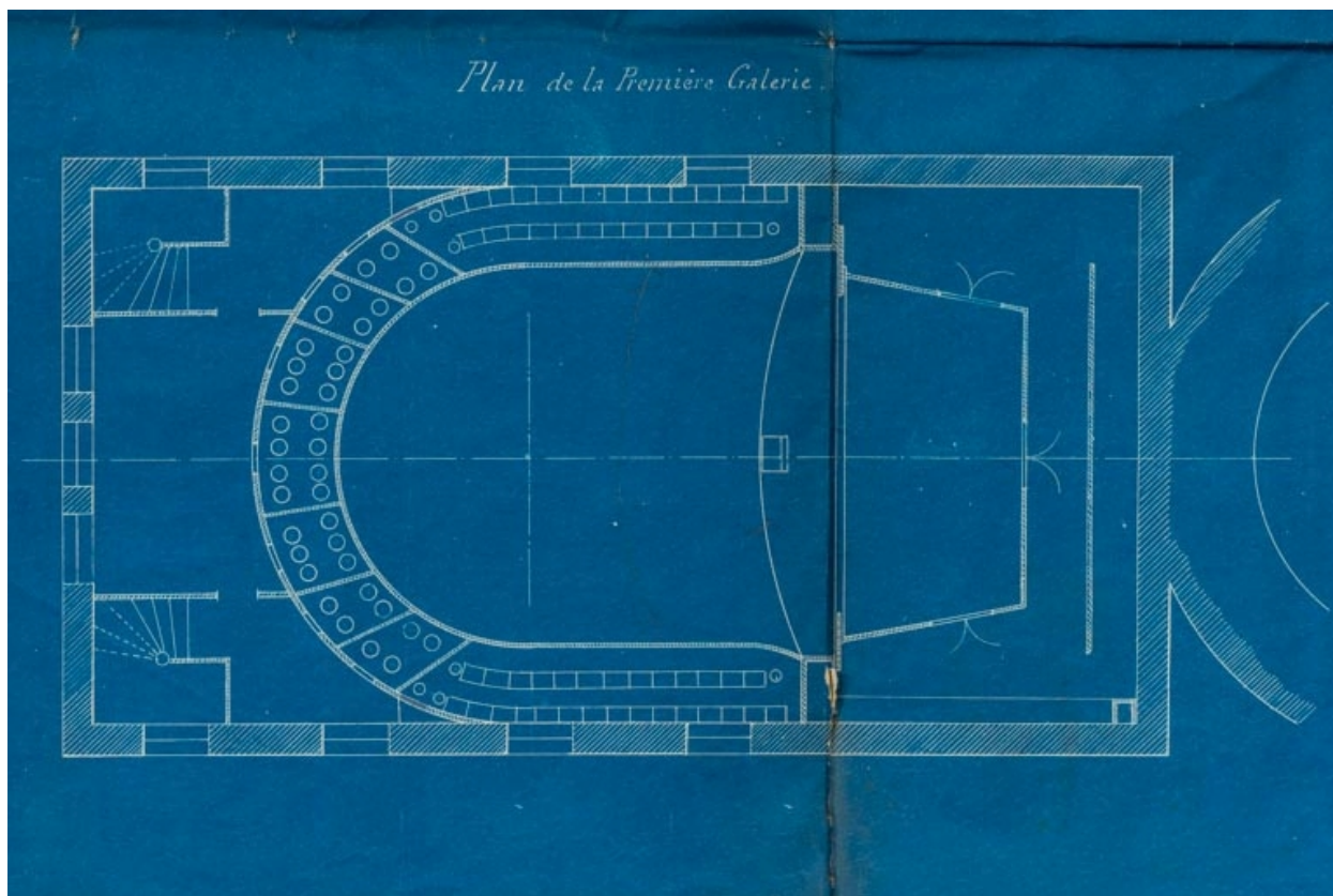
1721. Ville de Semur. Théâtre. Projet d'aménagement. [Détail :] Plan de la première galerie. S.d. [1903 ?].
