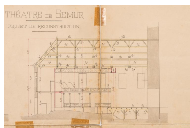
Théâtre de Semur. Projet de reconstruction. [Détail :] Coupe en long. 10 mai 1902. Phot. Pierre-Marie Barbe-Richaud, Autr. Hector Marcorelles IVR26_20222100256NUC4A
