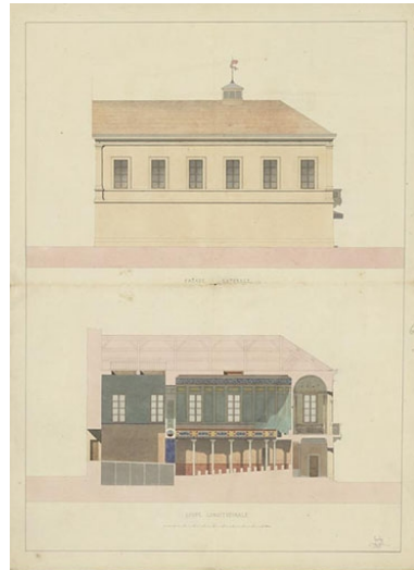
5. Façade latérale [et] 6. Coupe longitudinale. [Coupes et élévations par Grosley du théâtre projeté à Semur-en-Auxois]. S.d. [1843 ?]. Autr. Jean-Jacques Grosley IVR26_20222100280NUC2A
