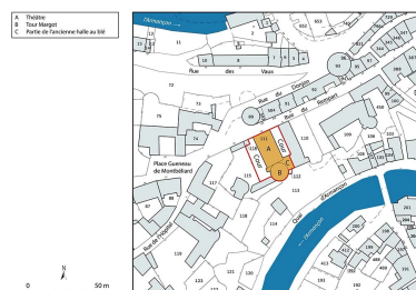
Plan-masse et de situation. Source : Direction générale des Finances Publiques - Cadastre ; mise à jour 2021, section AD, 1/1 000. Dess. Aline Thomas IVR26_20222100161NUDA
