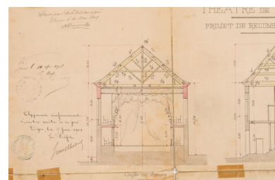
Théâtre de Semur. Projet de reconstruction. [Détail :] Coupe en travers. 10 mai 1902. Phot. Pierre-Marie Barbe-Richaud, Autr. Hector Marcorelles IVR26_20222100257NUC4A
