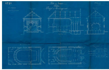
1721. Ville de Semur. Théâtre. Projet d'aménagement. S.d. [1903 ?]. Phot. Pierre-Marie Barbe-Richaud, Autr. Emile Wessbecher, Autr. Hector Marcorelles IVR26_20222100248NUC4A
