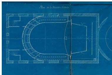
1721. Ville de Semur. Théâtre. Projet d'aménagement. [Détail :] Plan de la première galerie. S.d. [1903 ?]. Phot. Pierre-Marie Barbe-Richaud, Autr. Emile Wessbecher, Autr. Hector Marcorelles IVR26_20222100253NUC2A
