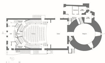
Plan au rez-de-chaussée. D'après un plan établi en 2019 par V.G. Dess. Aline Thomas IVR26_20222100166NUDA
