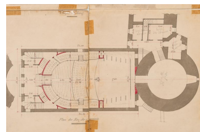
Théâtre de Semur. Projet de reconstruction. [Détail :] Plan du rez-de-chaussée. 10 mai 1902. Phot. Pierre-Marie Barbe-Richaud, Autr. Hector Marcorelles IVR26_20222100255NUC4A
