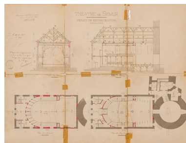
Théâtre de Semur. Projet de reconstruction. 10 mai 1902. Phot. Pierre-Marie Barbe-Richaud, Autr. Hector Marcorelles IVR26_20222100258NUC4A
