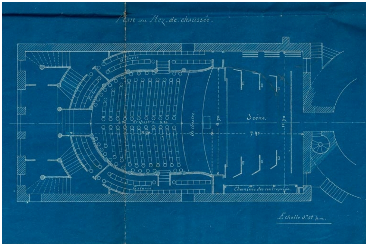
1721. Ville de Semur. Théâtre. Projet d'aménagement. [Détail :] Plan du rez-de-chaussée. S.d. [1903 ?].
