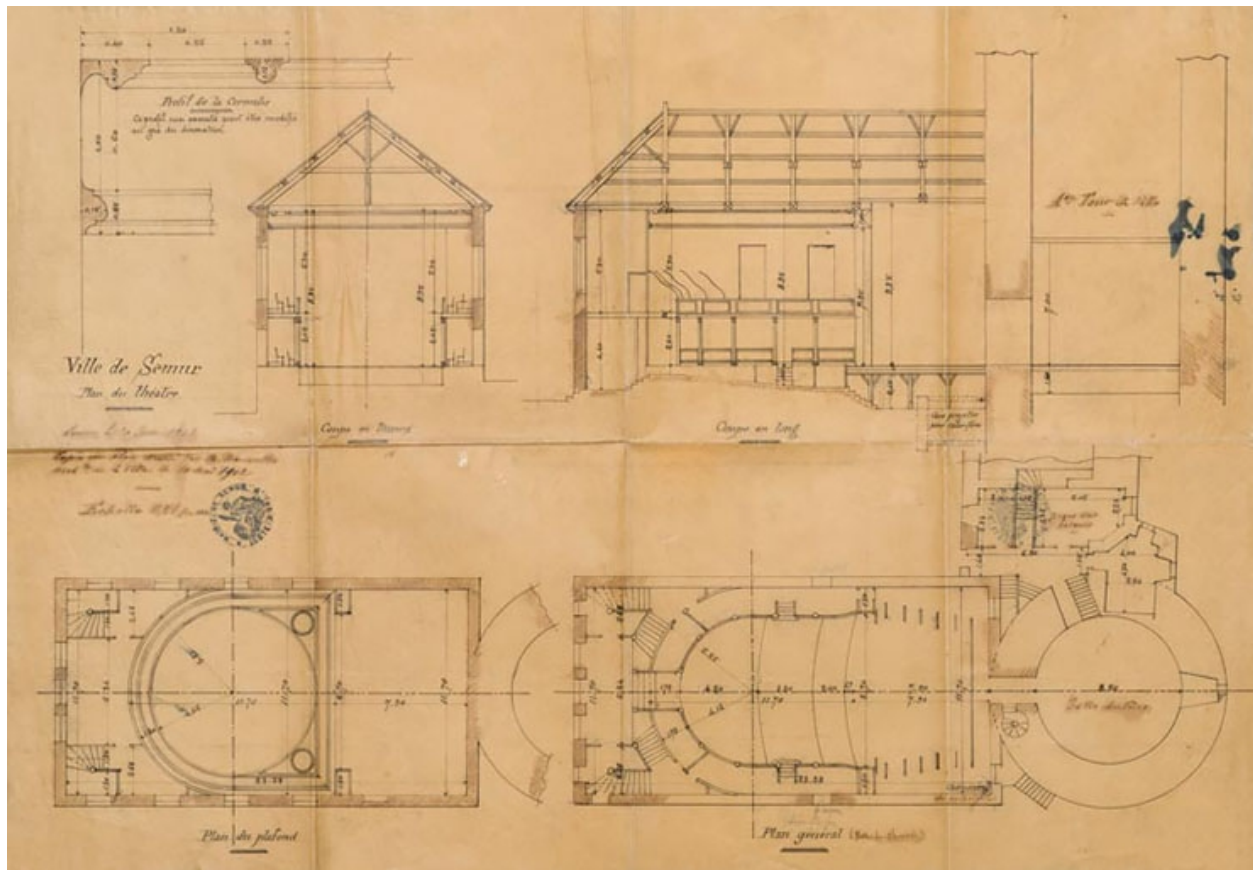
Ville de Semur. Plan du théâtre. 20 janvier 1903. Copie du plan dressé par M Marcorelles arch[itec]te de la Ville le 10 mai 1902.
