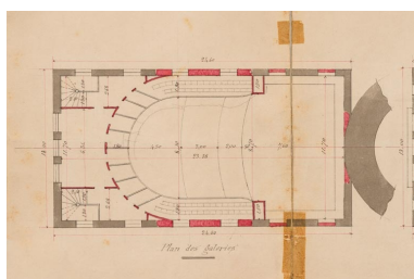
Théâtre de Semur. Projet de reconstruction. [Détail :] Plan des galeries. 10 mai 1902. Phot. Pierre-Marie Barbe-Richaud, Autr. Hector Marcorelles IVR26_20222100254NUC4A
