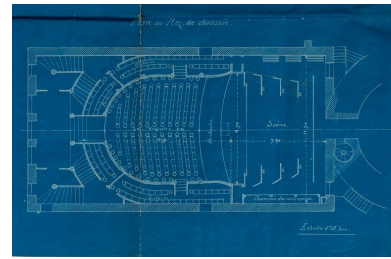
1721. Ville de Semur. Théâtre. Projet d'aménagement. [Détail :] Plan du rez-de-chaussée. S.d. [1903 ?]. Phot. Pierre-Marie Barbe-Richaud, Autr. Emile Wessbecher, Autr. Hector Marcorelles IVR26_20222100252NUC2A
