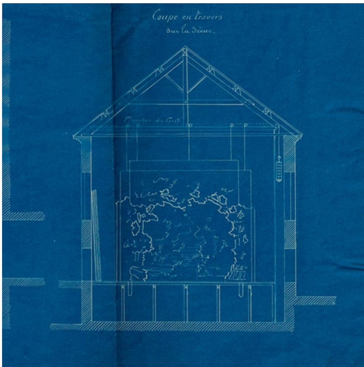
1721. Ville de Semur. Théâtre. Projet d'aménagement. [Détail :] Coupe en travers sur la scène. S.d. [1903 ?].
