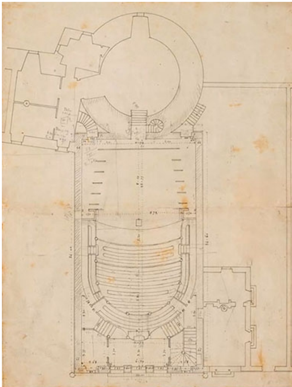
Dessin n° 5. Projet définitif d'un théâtre pour semur par Grosley sous la direction de Mr Bruzard [... Plan au rez-de-chaussée]. S.d. [1843 ?].
