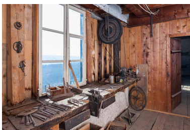
Ferme : établi et tour à bois à marchepied de l'atelier. Phot. Jérôme Mongreville IVR43_20142500266NUC4A
