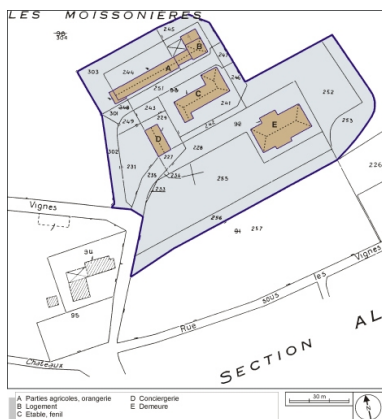
Plan-masse et de situation. Extrait du plan cadastral, 1984, section AK, 1:1000. Dess. André Céréza IVR43_20039000014NUDA
