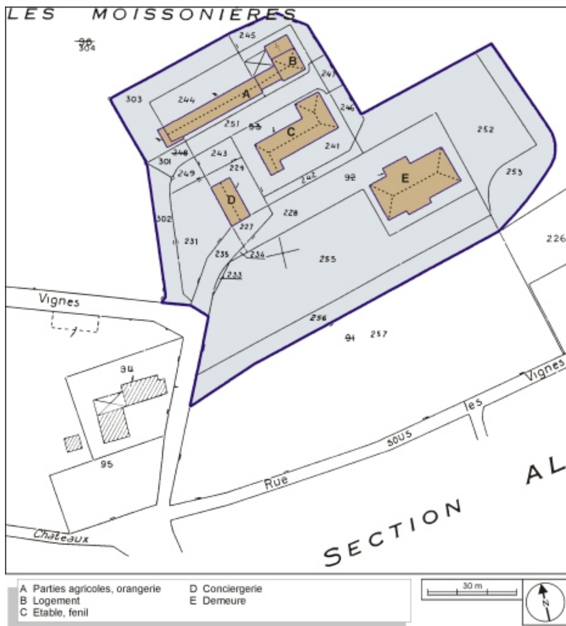
Plan-masse et de situation. Extrait du plan cadastral, 1984, section AK, 1:1000.
