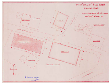
Etab[li]ssement]s "Elector" - "Securitor". Plan d'ensemble de situation. Bâtiments et abords [projet d'extension], 1954. Phot. Jérôme Mongreville, Autr. auteur inconnu IVR43_20132500591NUC4A
