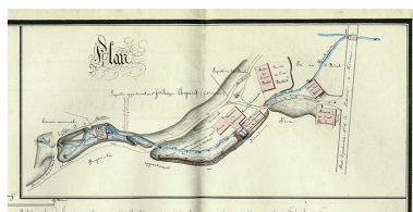
Plan et nivellements relatifs à la demande formée par le Sr François Philippe Chopard [...] tendant à obtenir l'autorisation d'établir une roue hydraulique à la brasserie [...] : détail], 11 mars 1844. Autr. Em. Raillard IVR43_20182500029NUC4A
