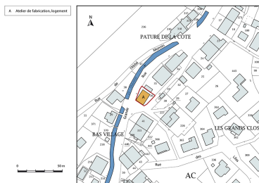
Plan-masse et de situation. Extrait du plan cadastral, 2017, section AC, 1/1 000. Dess. Mathias Papigny IVR43_20172501252NUDA
