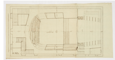
Plan de l'intérieur de la salle de spectacle d'Auxerre. Travaux. S.d. [an IX (1800-1801) ?]. Phot. Pierre-Marie Barbe- Richaud, Autr. Leblanc IVR26_20238900516NUC2A
