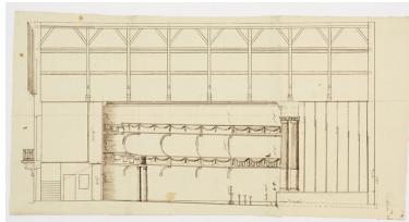
[Théâtre : coupe longitudinale]. S.d. [an IX (1800-1801) ?]. Phot. Pierre-Marie Barbe- Richaud, Autr. Leblanc IVR26_20238900515NUC2A
