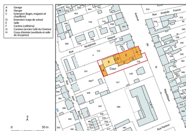
Plan-masse et de situation. Extrait du plan cadastral de la Direction Générale des Finances Publiques (DGFIP), 2022, section L, 1/1 000.
