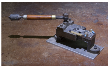
Machine à cintrer les nez, à coulisseau horizontal. Phot. Yves Sancey IVR43_20103900286NUC2A
