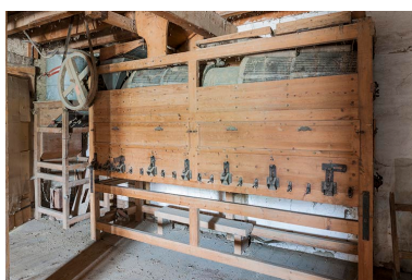
Trieur à grains Emile Marot.
