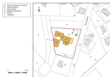
Plan-masse et de situation. Extrait du plan cadastral, 2016, section AE. Dess. Mathias Papigny IVR43_20162501766NUDA
