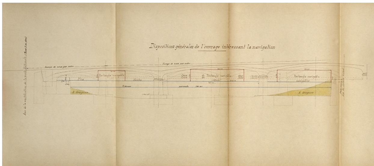
Projet de reconstruction du pont suspendu : dispositions générales de l'ouvrage intéressant la navigation (1912).
