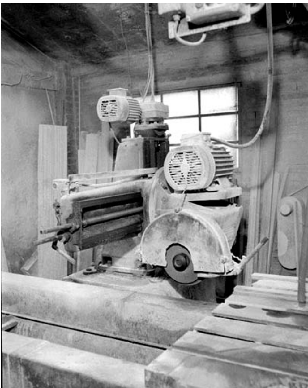
Débiteuse-moulineuse sud : bâti vertical, moteur et toupie.
