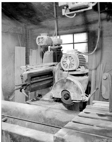
Débiteuse-moulreuse sud : bâti vertical, moteur et toupie. Phot. Yves Sancey IVR43_19933900345X
