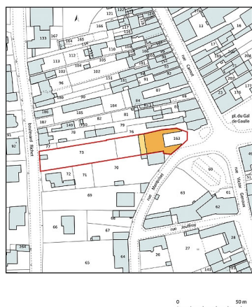
Plan-masse et de situation, extrait du plan cadastral (2021). Dess. Pierre-Marie Barbe-Richaud IVR43_20217000185NUDA
