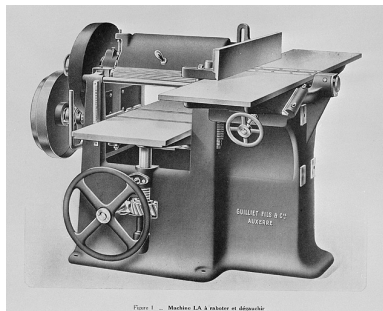
Machine LA à raboter et dégauchir. Phot. Yves Sancey IVR43_20022500918X
