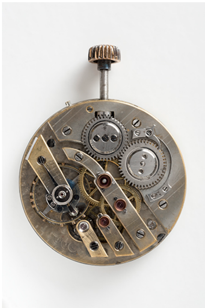
Mouvement Parrenin-Marguet : face côté ponts.
