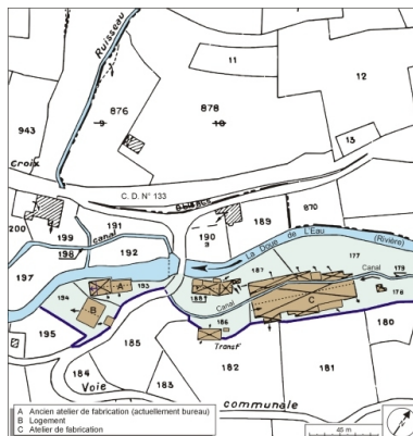
Plan-masse et de situation. Extrait du plan cadastral numérisé, 2005, section B, 1:2000 agrandi à 1:1500. Dess. André Céréza IVR43_20067000051NUDA
