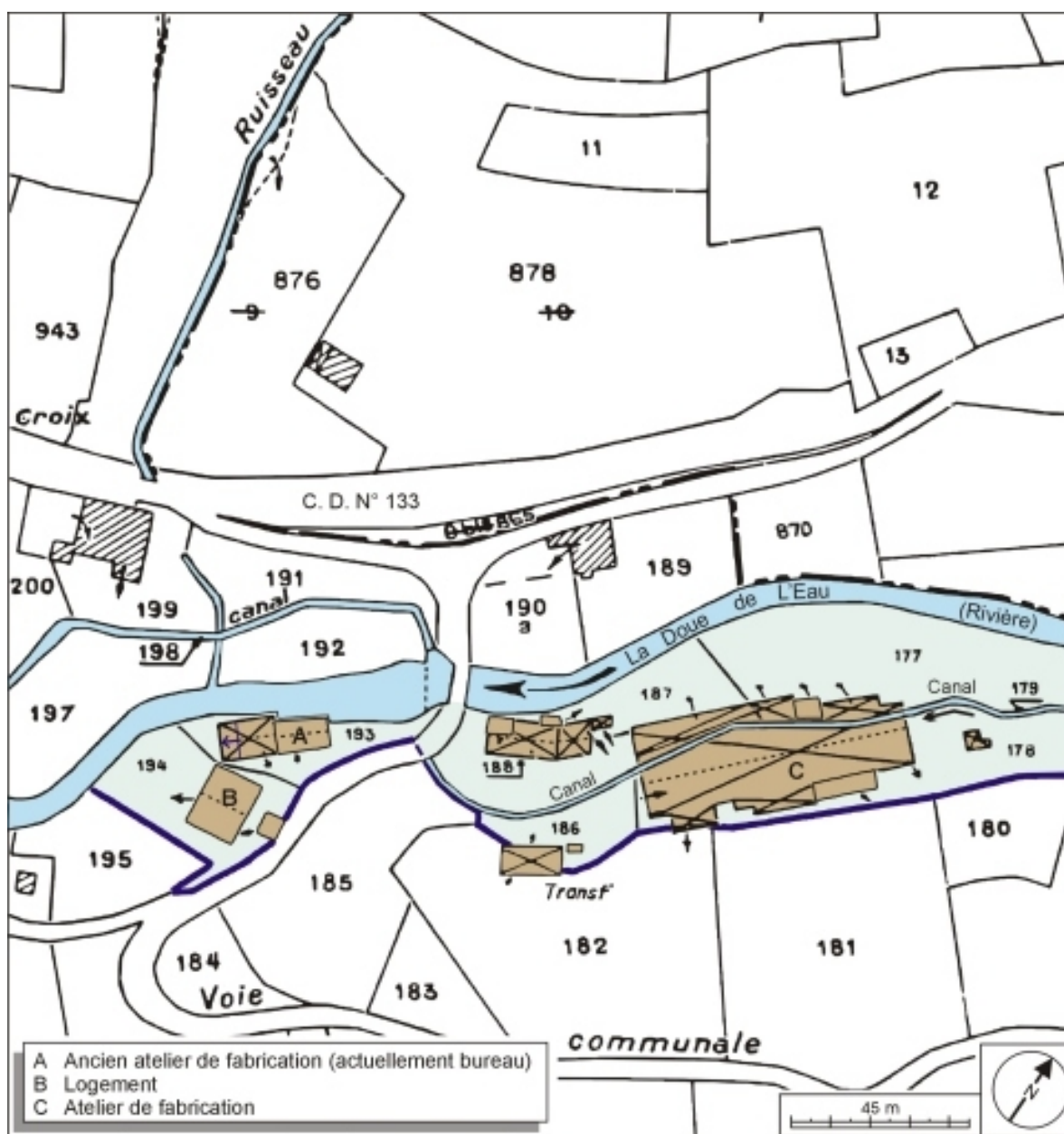
Plan-masse et de situation. Extrait du plan cadastral numérisé, 2005, section B, 1:2000 agrandi à 1:1500.
