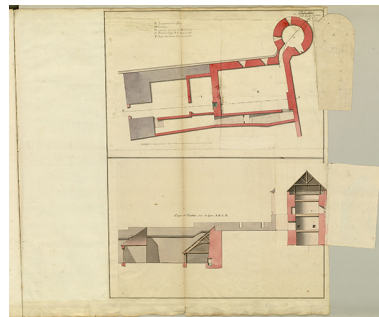
Folio 13. Ville de Salins. Tour ronde et cavalier de la porte Barbarine. N°2. Plan, coupe et élévation. Phot. auteur inconnu IVR43_20243900498NUC4A
