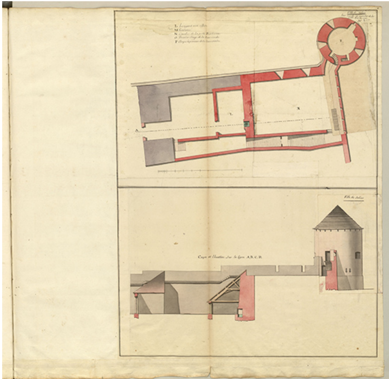
Folio 13. Ville de Salins. Tour ronde et cavalier de la porte Barbarine. N°2. Plan, coupe et élévation.
