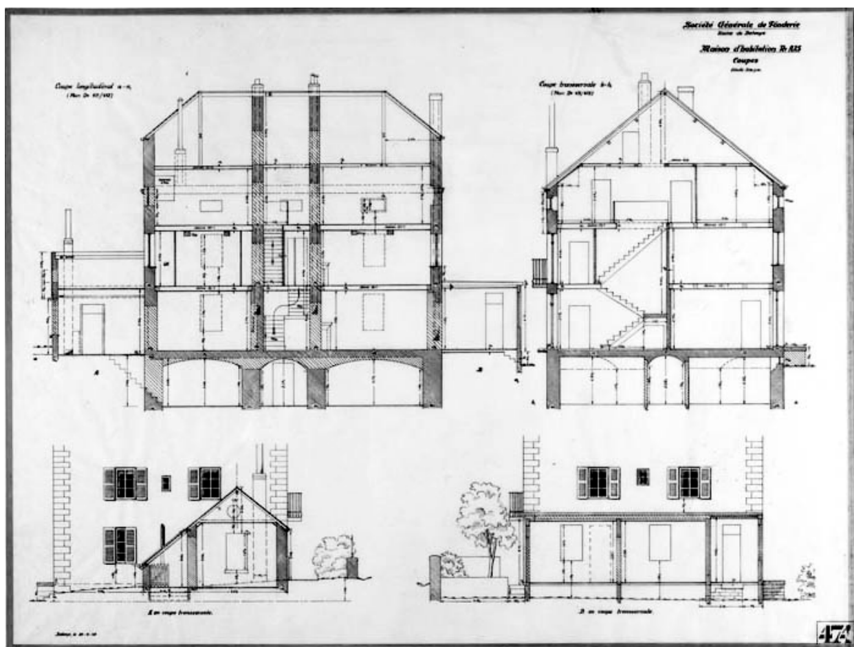
Société Générale de Fonderie. Usine de Belvoye. Maison d'habitation n° A25. Coupes.
