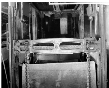
Guide support d'un châssis porte-lames. Phot. Yves Sancey IVR43_19933900284X
