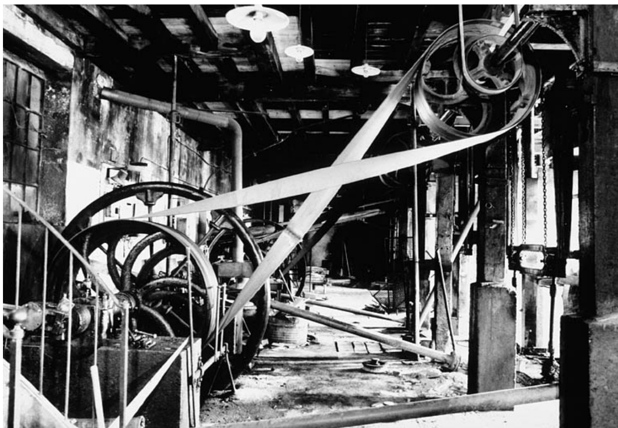
Système d'entraînement : côté transmission. Manivelle et volant d'inertie à droite, bielle au centre.
