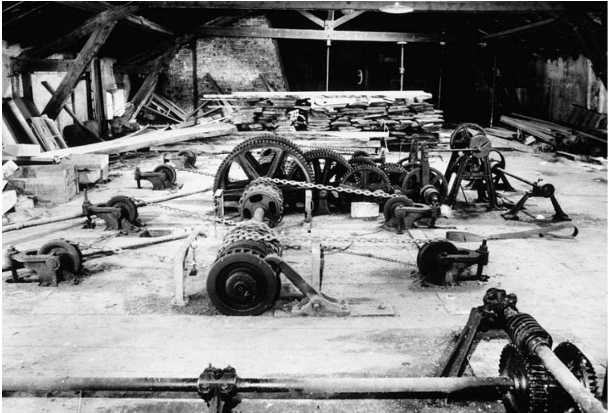
Système de descente à chaînes (châssis 1 et 2).
