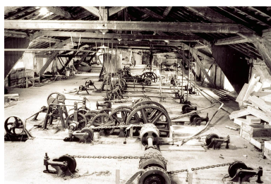
Système de descente des châssis porte-lames.
