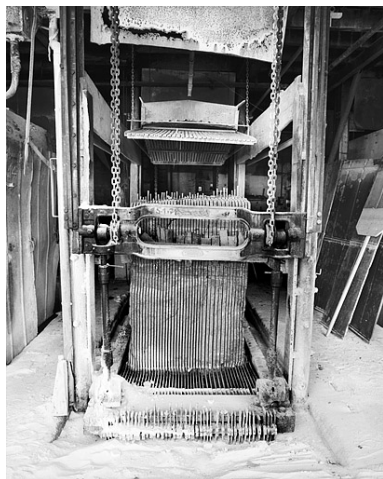
Scie Décamps, vue de face. Phot. Yves Sancey IVR43_19933900278X
