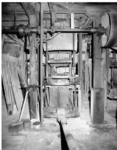
Système d'entraînement : côté châssis porte-lames. Transmission au plafond, extrémité de la bielle visible au centre. Phot. Yves Sancey IVR43_19933900287X
