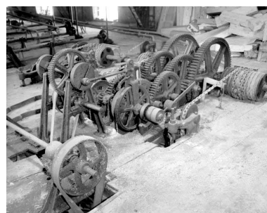
Système de descente à chaînes : détail.
