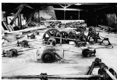
Système de descente à chaînes (châssis 1 et 2).
