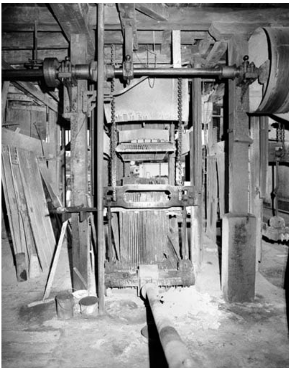
Système d'entraînement : côté châssis porte-lames. Transmission au plafond, extrémité de la bielle visible au centre.
