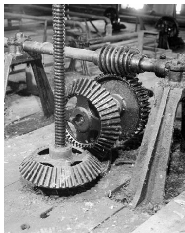
Système de descente à vis : détail.
