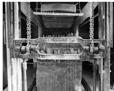
Guide support du châssis porte- lames d'une scie Décamps. Phot. Yves Sancey IVR43_19933900282X
