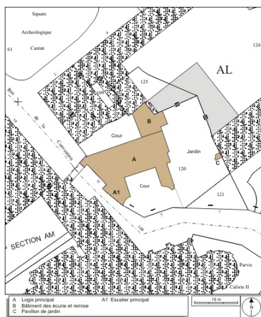
Plan masse et de situation. Extrait du plan cadastral, 1974, section AL. Dess. André Céréza IVR43_20092501212NUDA
