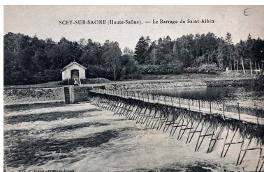
Le barrage à aiguilles de Saint-Albin, carte postale. Phot. Jérôme Mongreville, Autr. auteur inconnu IVR43_20197000066NUC4A
