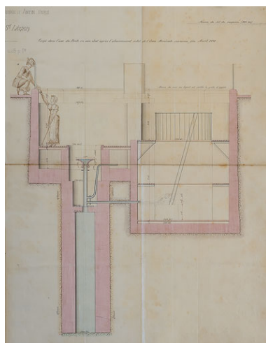
Coupe sur les deux puits avant et après l'abaissement du niveau de l'eau survenu fin avril 1891, détail de l'état postérieur. Phot. Pierre-Marie Barbe-Richaud, Autr. auteur inconnu IVR26_20205800311NUC2A
