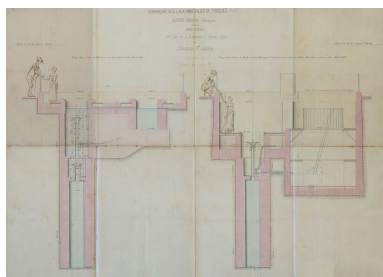
Coupe sur les deux puits avant et après l'abaissement du niveau de l'eau survenu fin avril 1891. Phot. Pierre-Marie Barbe- Richaud, Autr. auteur inconnu IVR26_20205800309NUC4A
