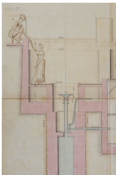
Coupe sur les deux puits avant et après l'abaissement du niveau de l'eau survenu fin avril 1891, détail de l'état postérieur. Phot. Pierre-Marie Barbe-Richaud, Autr. auteur inconnu IVR26_20205800312NUC4A
