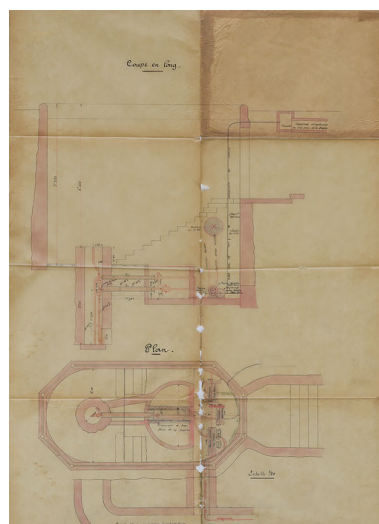
Installation d'un système de pompage dans la nouvelle chambre de captage (1904). Phot. Pierre-Marie Barbe-Richaud, Autr. auteur inconnu IVR26_20205800191NUC4A
