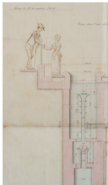
Coupe sur les deux puits avant et après l'abaissement du niveau de l'eau survenu fin avril 1891, détail de l'état antérieur. Phot. Pierre-Marie Barbe- Richaud, Autr. auteur inconnu IVR26_20205800313NUC4A
