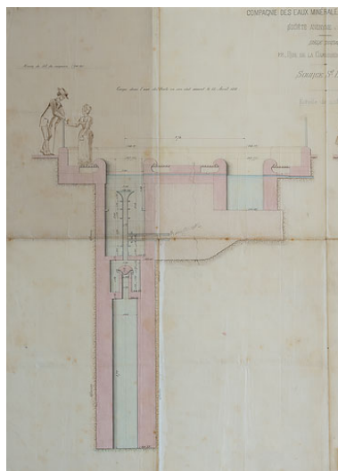
Coupe sur les deux puits avant et après l'abaissement du niveau de l'eau survenu fin avril 1891, détail de l'état antérieur. Phot. Pierre-Marie Barbe- Richaud, Autr. auteur inconnu IVR26_20205800310NUC4A
