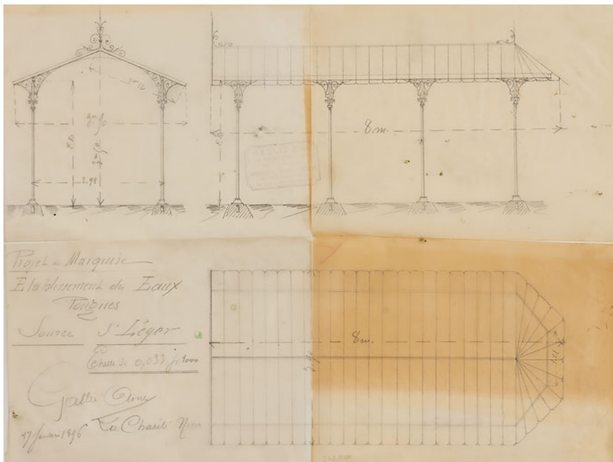
Projet de marquise (1896) par Gallié Aîné.
