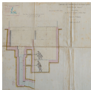
Coupe sur les deux puits montrant le niveau de l'eau à la fin de l'année 1891. Phot. Pierre-Marie Barbe-Richaud, Autr. auteur inconnu IVR26_20205800308NUC2A
