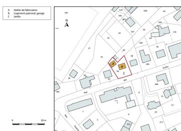
Plan-masse et de situation. Extrait du plan cadastral, 2013, section AB. Dess. Mathias Papigny IVR43_20142501524NUDA
