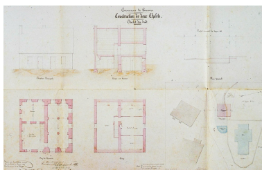
Commune de Lamarre. Construction de deux chalets. Chalet du sud : plan, coupes et élévation. Phot. Dominique Dominguez, Autr. Achille Paillot IVR43_19813900306XA
