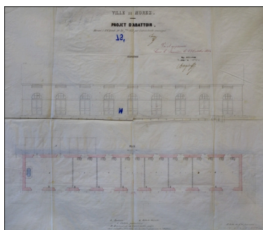
Ville de Morez. Projet d'abattoir. Plan [et] Elévation, 1852. Phot. Yves Sancey, Autr. Comoy IVR43_20103900062NUC2A
