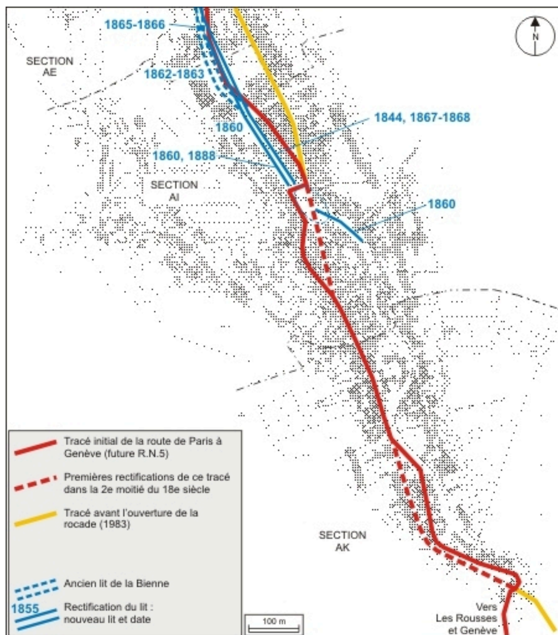
Plan des rectifications du tracé de la route de Paris à Genève et du cours de la Bienne : partie sud. Montage de feuilles cadastrales, 1980, sections AE, AI et AK, échelle 1:1000 réduite à 1:6000.
