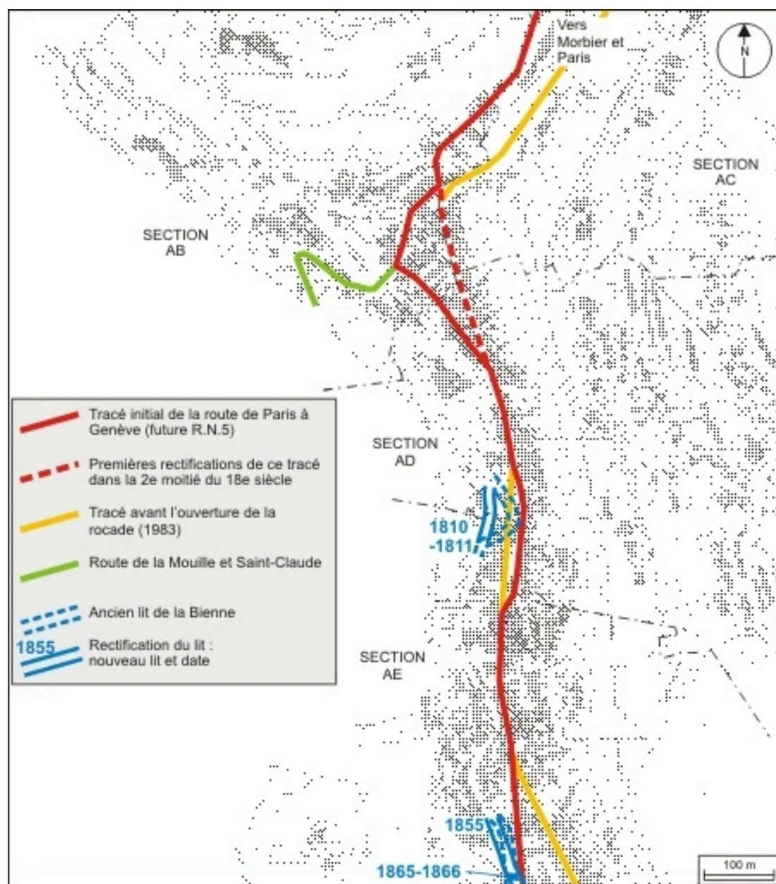
Plan des rectifications du tracé de la route de Paris à Genève et du cours de la Bienne : partie nord. Montage de feuilles cadastrales, 1980, sections AB, AC, AD et AE, échelle 1:1000 réduite à 1:6000.
