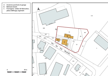
Plan-masse et de situation. Extrait du plan cadastral, 2018, section AB. Dess. Bertrand Turina IVR43_20202500307NUDA
