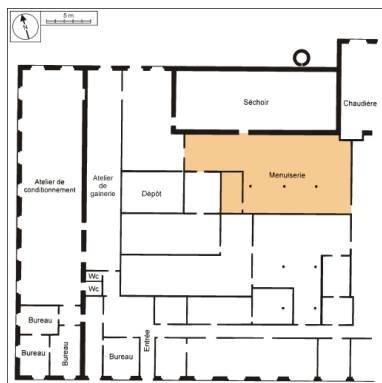
Plan de situation de l'atelier de menuiserie. Dess. André Céréza IVR43_20022501335NUDA
