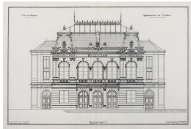
Ville de Nevers. Restauration du Théâtre. Façade principale [projet de façade avec porche, encadré par deux pavillons, et toit brisé]. 1er avril 1898. Phot. Pierre-Marie Barbe-Richaud, Autr. Charles Brazeau IVR26_20245800416NUC4A
