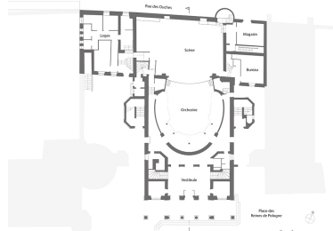
Plan au rez-de-chaussée. D'après un plan de 2018 du géomètre Xavier de Taillandier, fourni par la Ville de Nevers. Dess. Aline Thomas IVR26_20255800002NUDA
