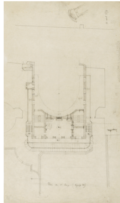
[Projet avec marquise, balcons et escaliers extérieurs]. Plan du 1er étage (Foyer et 2es). S.d. [1894]. Phot. Pierre-Marie Barbe-Richaud, Autr. Charles Brazeau IVR26_20245800422NUC2A
