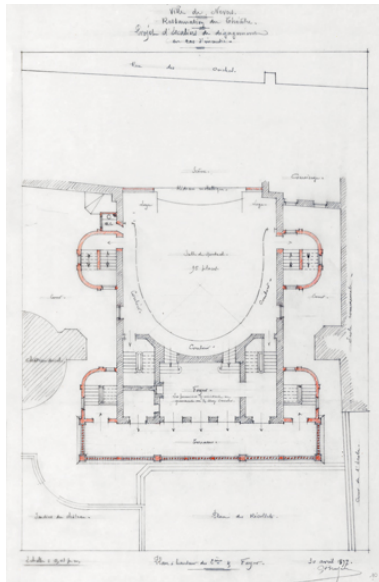
Restauration du Théâtre. Projet d'escaliers de dégagement en cas d'incendie. Plan des 2èmes et Foyer. 30 avril 1897. Phot. Pierre-Marie Barbe-Richaud, Autr. Charles Brazeau IVR26_20245800435NUC4A
