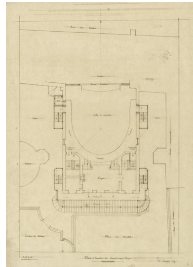
Théâtre. Projet de marquise vitrée et d'escaliers extérieurs. Plan à hauteur des Deuxièmes et Foyer. 20 janvier 1897. Phot. Pierre-Marie Barbe-Richaud, Autr. Charles Brazeau IVR26_20245800427NUC4A
