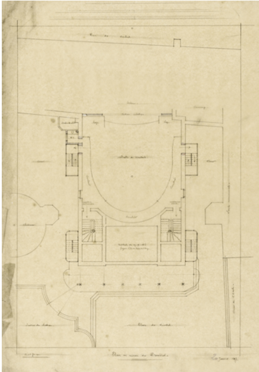
Théâtre. Projet de marquise vitrée et d'escaliers extérieurs. Plan au niveau des Premières. 20 janvier 1897.
