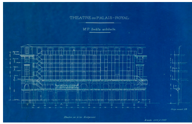
Théâtre du Palais Royal. M Sédille, architecte. S.d. [décennie 1880]. Phot. Pierre-Marie Barbe-Richaud, Autr. Paul Sédille IVR26_20245800441NUC4A
