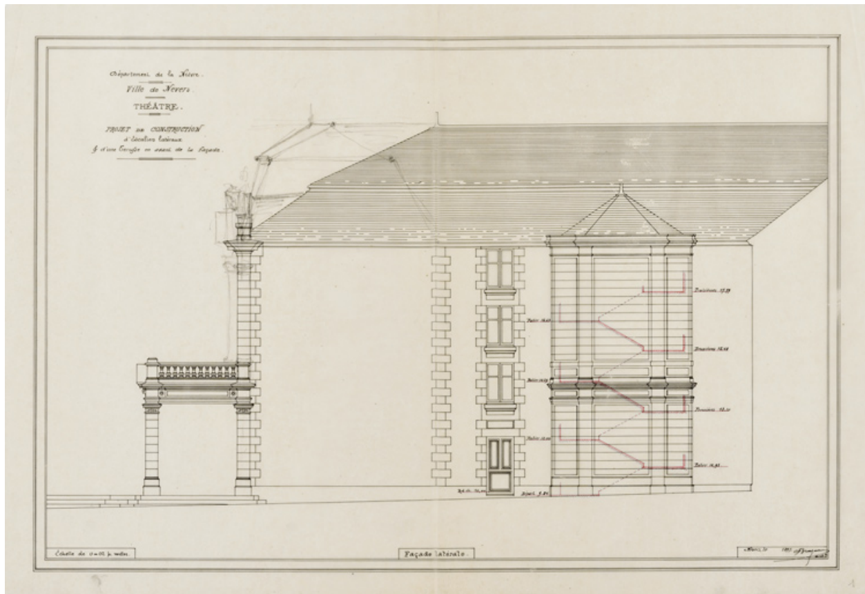
Théâtre. Projet de construction d'escaliers latéraux et d'une terrasse en avant de la façade. Façade latérale [droite]. [Mai-juin] 1897.
