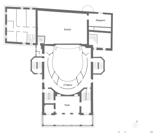
Plan au 2e étage. D'après un plan de 2018 du géomètre Xavier de Taillandier, fourni par la Ville de Nevers. Dess. Aline Thomas IVR26_20255800003NUDA
