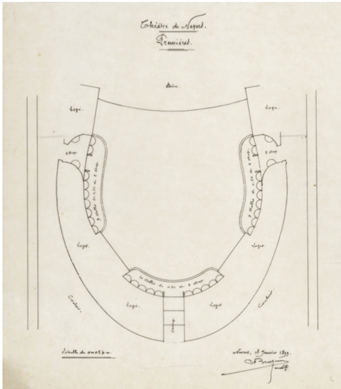
Théâtre de Nevers [implantation des loges et des sièges]. Premières. 18 janvier 1899.
