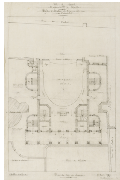
Restauration du Théâtre. Projet d'escaliers de dégagement en cas d'incendie. Plan du Rez-de-chaussée. 30 avril 1897. Phot. Pierre-Marie Barbe-Richaud, Autr. Charles Brazeau IVR26_20245800434NUC4A
