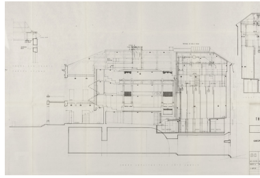
Ville de Nevers. Théâtre municipal. Mise en conformité. 6B. Coupe longitudinale. 1976. Phot. Pierre-Marie Barbe-Richaud, Autr. Camille Demangeat, Autr. Michel Rioualec IVR26_20245800469NUC4A
