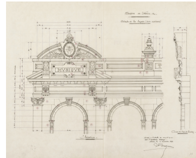
Théâtre de Nevers. Détails de la façade (partie supérieure). 10 décembre 1898. Phot. Pierre-Marie Barbe-Richaud, Autr. Charles Brazeau IVR26_20245800418NUC2A
