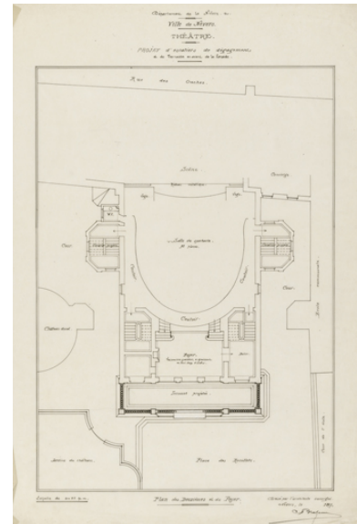
Théâtre. Projet d'escaliers de dégagement et de terrasse en avant de la façade. Plan des Deuxièmes et du Foyer. [Mai-juin] 1897. Phot. Pierre-Marie Barbe-Richaud, Autr. Charles Brazeau IVR26_20245800433NUC4A
