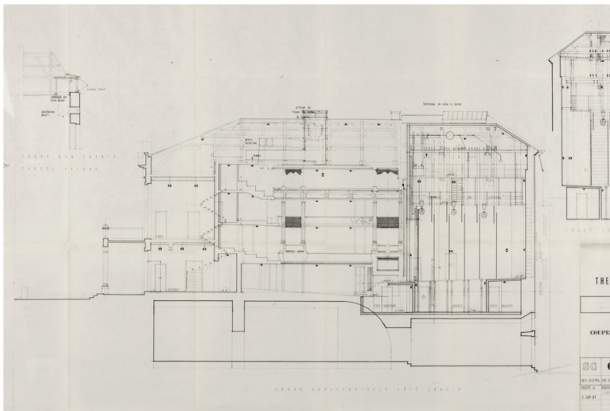
Ville de Nevers. Théâtre municipal. Mise en conformité. 6B. Coupe longitudinale. 1976.
