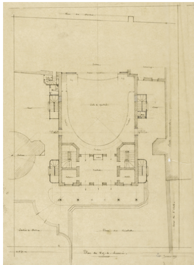
Théâtre. Projet de marquise vitrée et d'escaliers extérieurs. Plan du Rez-de-chaussée. 20 janvier 1897. Phot. Pierre-Marie Barbe-Richaud, Autr. Charles Brazeau IVR26_20245800430NUC2A
