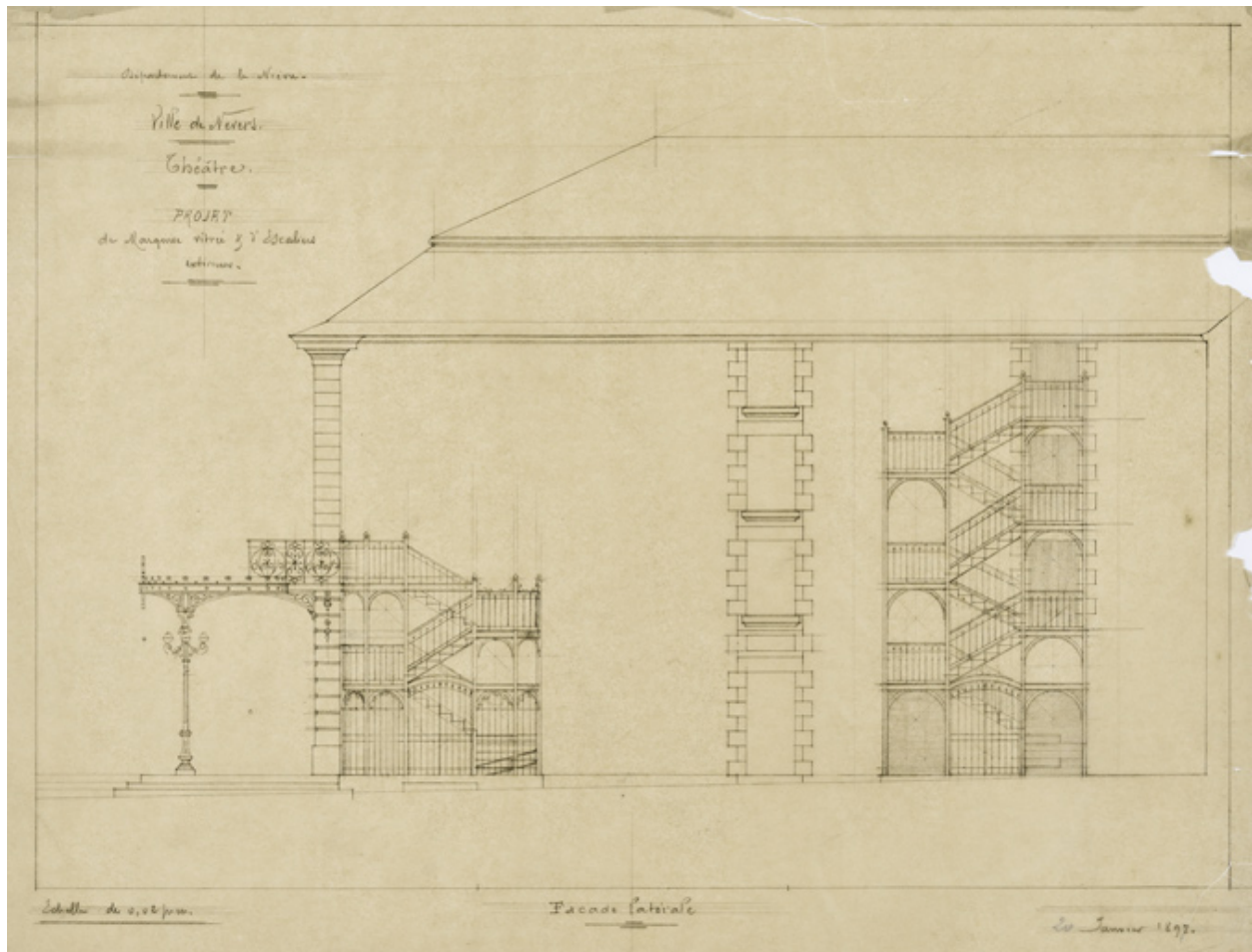
Théâtre. Projet de marquise vitrée et d'escaliers extérieurs. Façade latérale. 20 janvier 1897.
