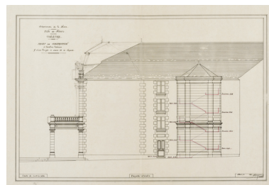
Théâtre. Projet de construction d'escaliers latéraux et d'une terrasse en avant de la façade. Façade latérale [droite]. [Mai-juin] 1897. Phot. Pierre-Marie Barbe-Richaud, Autr. Charles Brazeau IVR26_20245800412NUC4A
