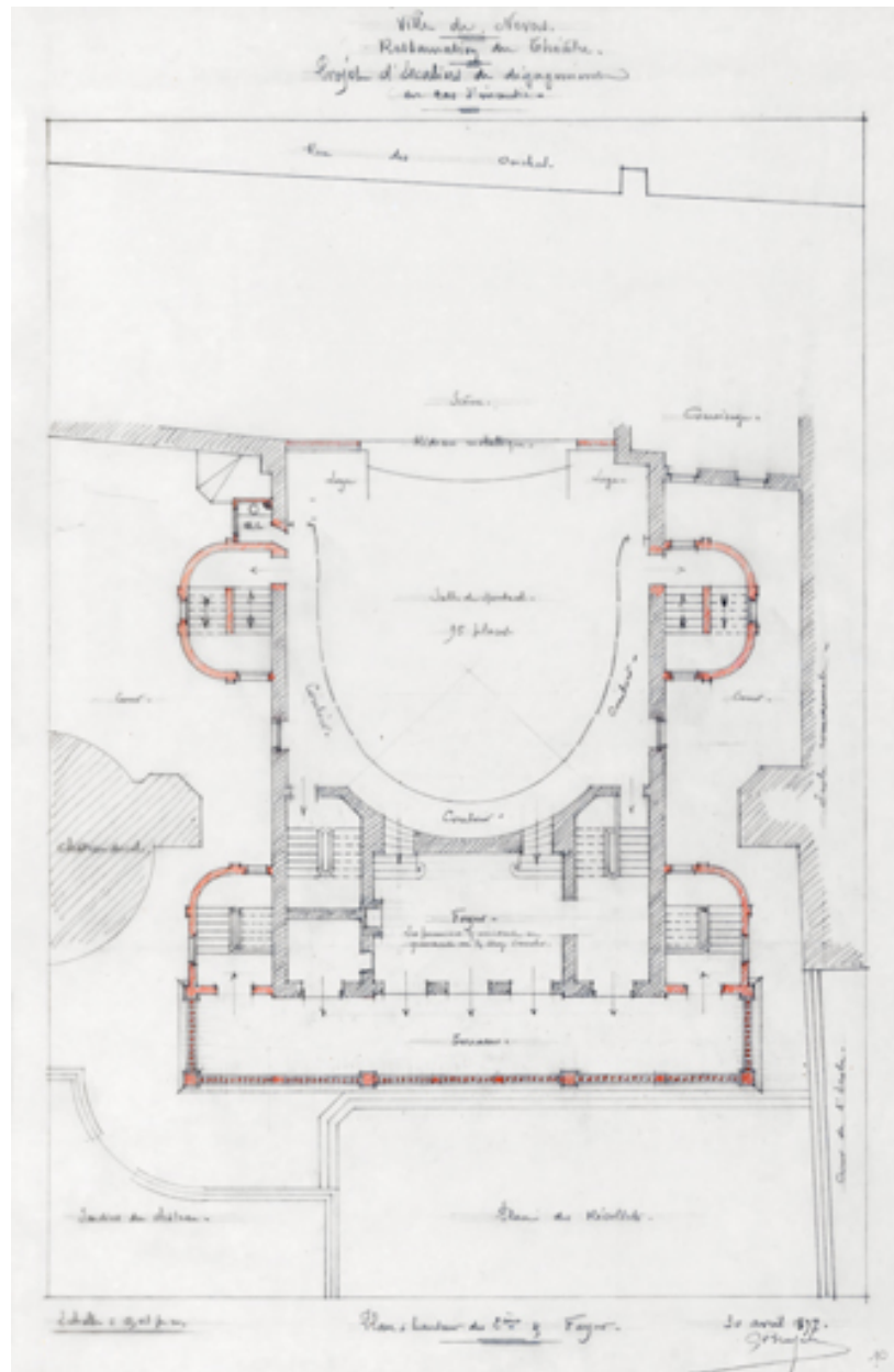
Restauration du Théâtre. Projet d'escaliers de dégagement en cas d'incendie. Plan des 2èmes et Foyer. 30 avril 1897.
