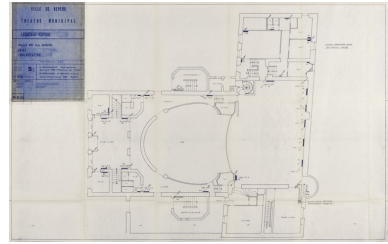
Ville de Nevers. Théâtre municipal. Chauffage central. SC 2. Implantation. Plan de la scène. Loges. Octobre 1978. Phot. Pierre-Marie Barbe-Richaud, Autr. Camille Demangeat, Autr. Michel Rioualec IVR26_20245800471NUC4A
