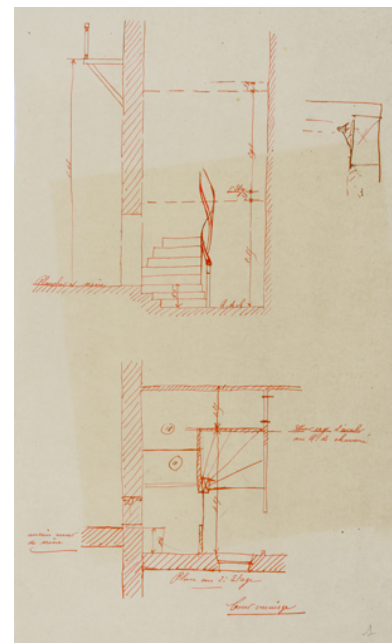
[Croquis de plan et coupe de l'escalier pour le concierge]. S.d. [1898 ?]. Phot. Pierre-Marie Barbe-Richaud, Autr. Charles Brazeau IVR26_20245800436NUC2A
