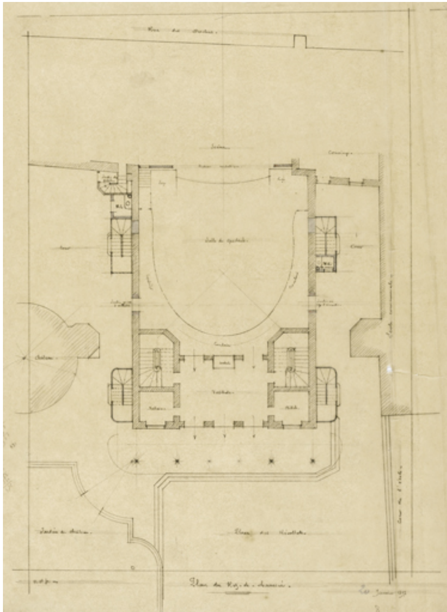
Théâtre. Projet de marquise vitrée et d'escaliers extérieurs. Plan du Rez-de-chaussée. 20 janvier 1897.
