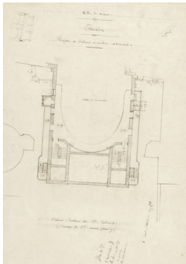
[Projet avec marquise, balcons et escaliers extérieurs]. Balcons à hauteur des 3es galeries (à hauteur des 1res même plan). S.d. [1894]. Phot. Pierre-Marie Barbe-Richaud, Autr. Charles Brazeau IVR26_20245800421NUC4A
