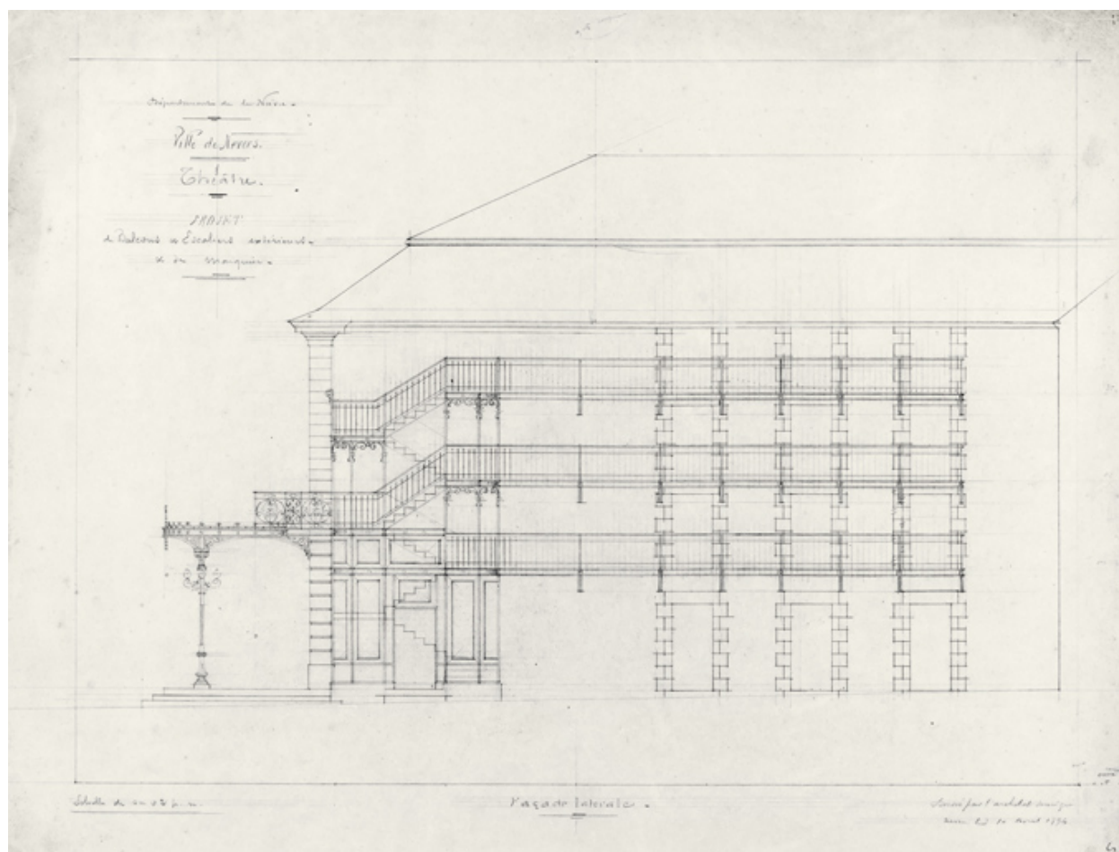
Ville de Nevers. Théâtre. Projet de balcons et escaliers extérieurs et de marquise. Façade latérale. 10 avril 1894.
