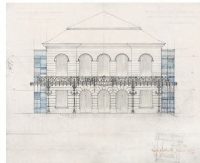
[Projet de façade avec marquise et escaliers latéraux]. 10 avril 1894 modifié le 20 janvier 1897. Phot. Pierre-Marie Barbe-Richaud, Autr. Charles Brazeau IVR26_20245800420NUC2A
