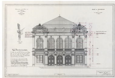
Ville de Nevers. Théâtre. Projet de restauration de la façade principale. Elévation [avec porche et toit brisé]. Septembre 1898. Phot. Pierre-Marie Barbe-Richaud, Autr. Charles Brazeau IVR26_20245800417NUC4A
