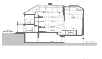
Coupe longitudinale. D'après une coupe de 2018 du géomètre Xavier de Taillandier, fournie par la Ville de Nevers. Dess. Aline Thomas IVR26_20255800004NUDA
