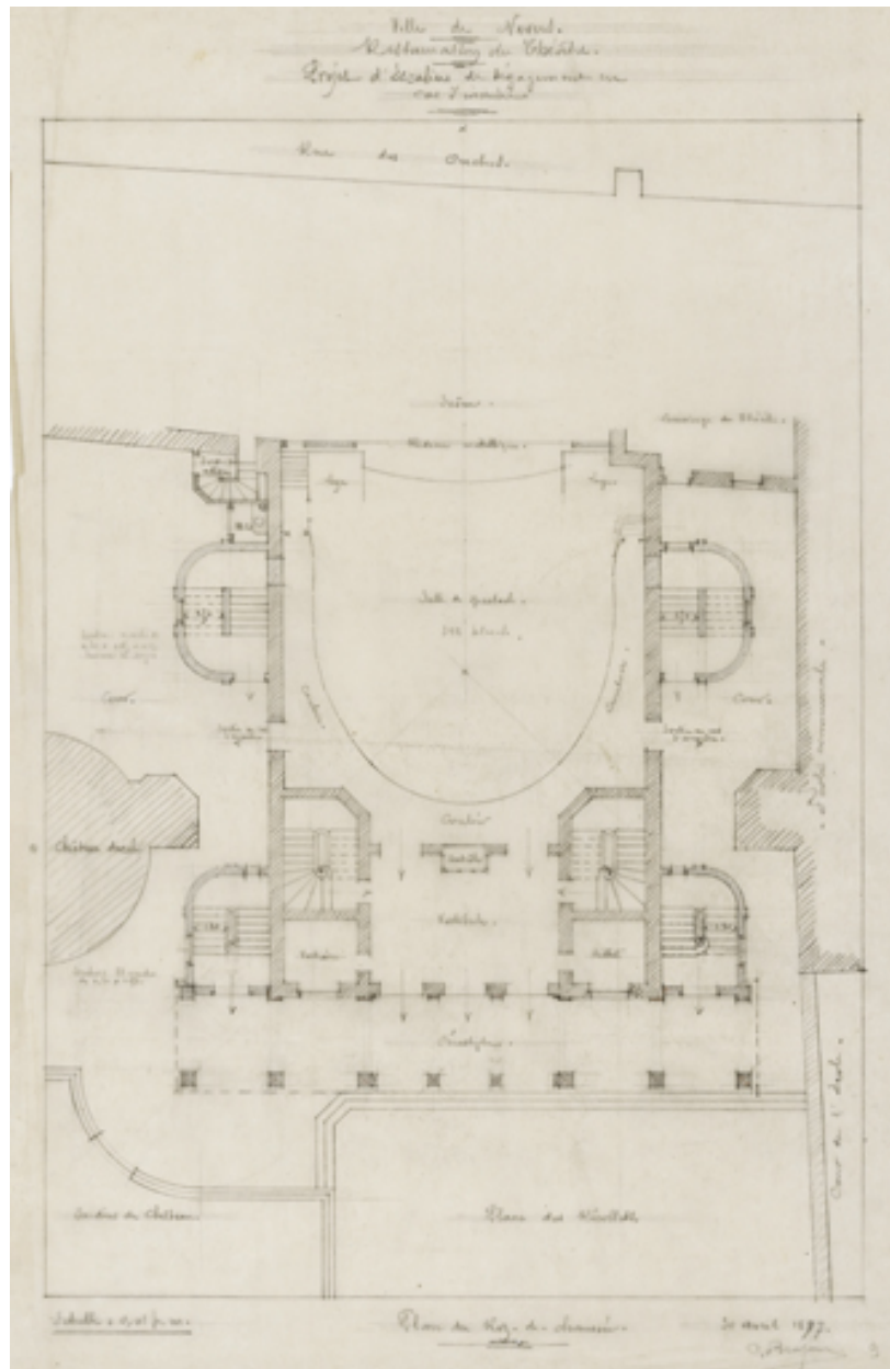
Restauration du Théâtre. Projet d'escaliers de dégagement en cas d'incendie. Plan du Rez-de-chaussée. 30 avril 1897.
