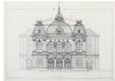
[Projet de façade avec porche, encadré par deux pavillons, et dôme carré]. S.d. [fin 1897 ou début 1898]. Phot. Pierre-Marie Barbe-Richaud, Autr. Charles Brazeau IVR26_20245800415NUC4A
