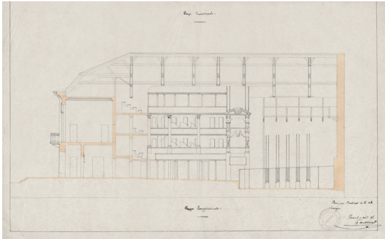
Projet de restauration de la salle de spectacle de la ville de Nevers. Coupe longitudinale. 9 avril 1851.
