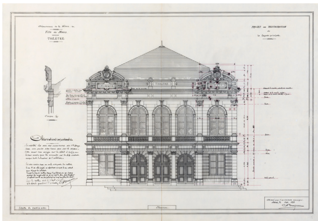
Ville de Nevers. Théâtre. Projet de restauration de la façade principale. Elévation [avec porche et toit brisé]. Septembre 1898.
