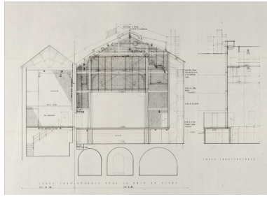
Ville de Nevers. Théâtre municipal. Mise en conformité. 1A. [Détail :] Coupe transversale sur baie de scène. 1976. Phot. Pierre-Marie Barbe-Richaud, Autr. Camille Demangeat, Autr. Michel Rioualec IVR26_20245800468NUC4A
