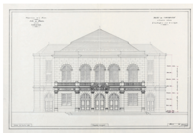
Théâtre. Projet de construction d'escaliers latéraux et d'une terrasse en avant de la façade. Façade principale. [Mai-juin] 1897. Phot. Pierre-Marie Barbe-Richaud, Autr. Charles Brazeau IVR26_20245800419NUC4A
