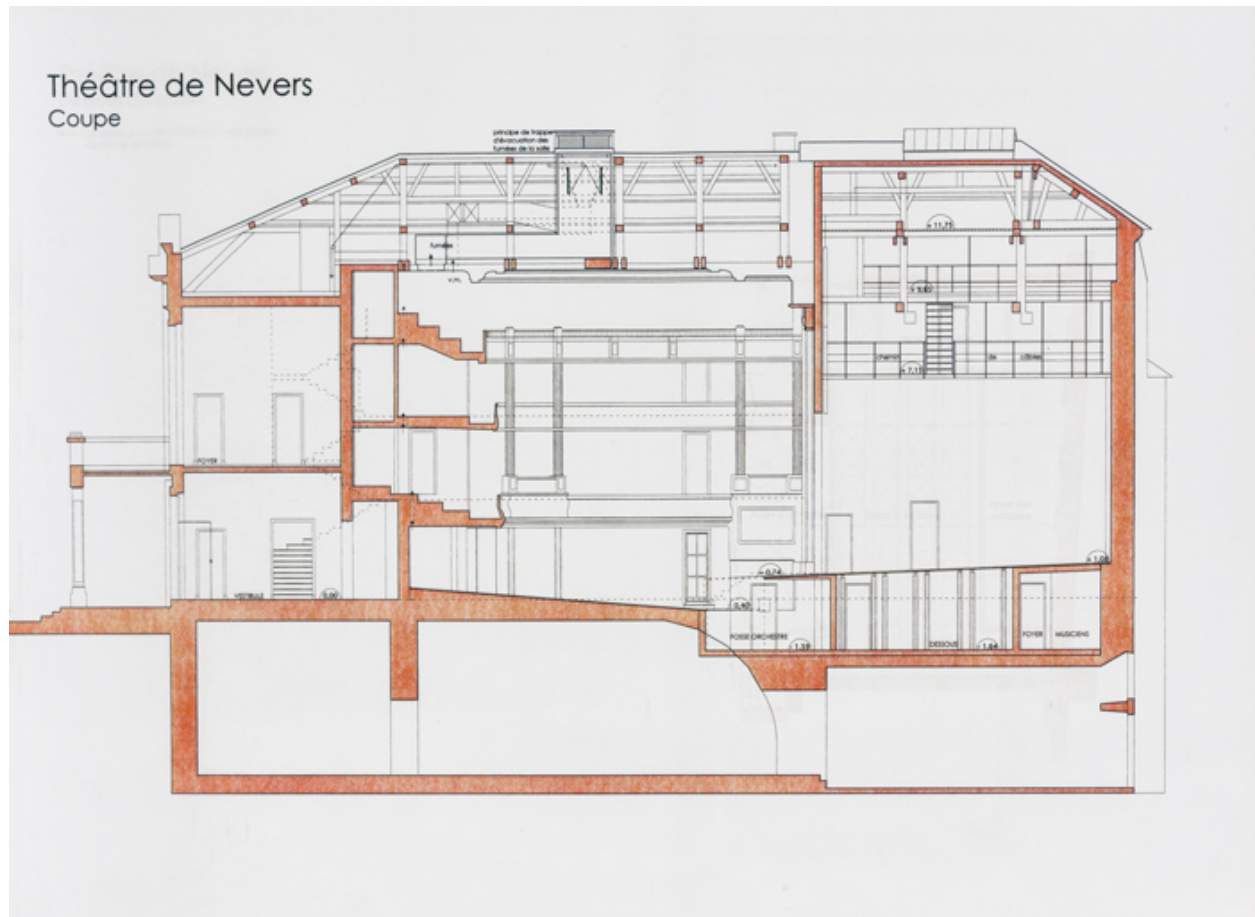
Théâtre de Nevers. Etat des lieux. Coupe. S.d. [octobre 2005].
