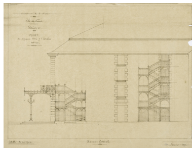
Théâtre. Projet de marquise vitrée et d'escaliers extérieurs. Façade latérale. 20 janvier 1897. Phot. Pierre-Marie Barbe-Richaud, Autr. Charles Brazeau IVR26_20245800431NUC2A
