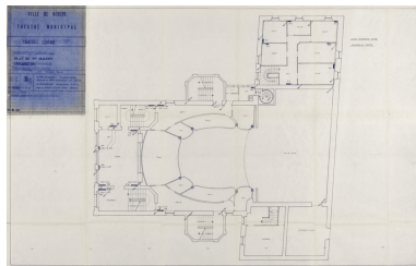
Ville de Nevers. Théâtre municipal. Chauffage central. SC 3. Implantation. Plan du 1er balcon. Octobre 1978. Phot. Pierre-Marie Barbe-Richaud, Autr. Camille Demangeat, Autr. Michel Rioualec IVR26_20245800470NUC4A
