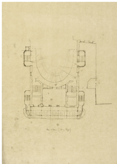
Théâtre. Projet de marquise vitrée et d'escaliers extérieurs. Plan à hauteur des Deuxièmes et Foyer [croquis]. 20 janvier 1897. Phot. Pierre-Marie Barbe-Richaud, Autr. Charles Brazeau IVR26_20245800428NUC2A
