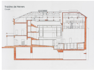
Théâtre de Nevers. Etat des lieux. Coupe. S.d. [octobre 2005]. Phot. Pierre-Marie Barbe-Richaud, Autr. auteur inconnu IVR26_20245800474NUC2A
