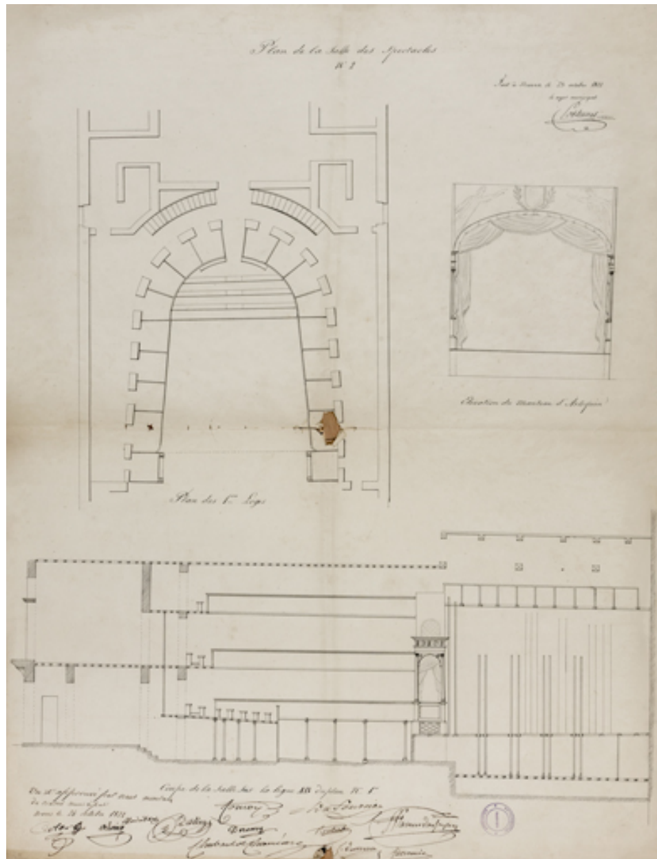
Plan de la salle des spectacles. N° 2. Plan des 1ères loges, Coupe de la salle sur la ligne AB du plan N° 1er [et] Elévation du Manteau d'Arlequin. 23 octobre 1822.
