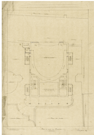
Théâtre. Projet de marquise vitrée et d'escaliers extérieurs. Plan au niveau des Premières. 20 janvier 1897. Phot. Pierre-Marie Barbe-Richaud, Autr. Charles Brazeau IVR26_20245800429NUC2A
