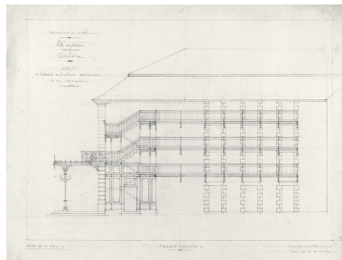
Ville de Nevers. Théâtre. Projet de balcons et escaliers extérieurs et de marquise. Façade latérale. 10 avril 1894. Phot. Pierre-Marie Barbe-Richaud, Autr. Charles Brazeau IVR26_20245800423NUC4A
