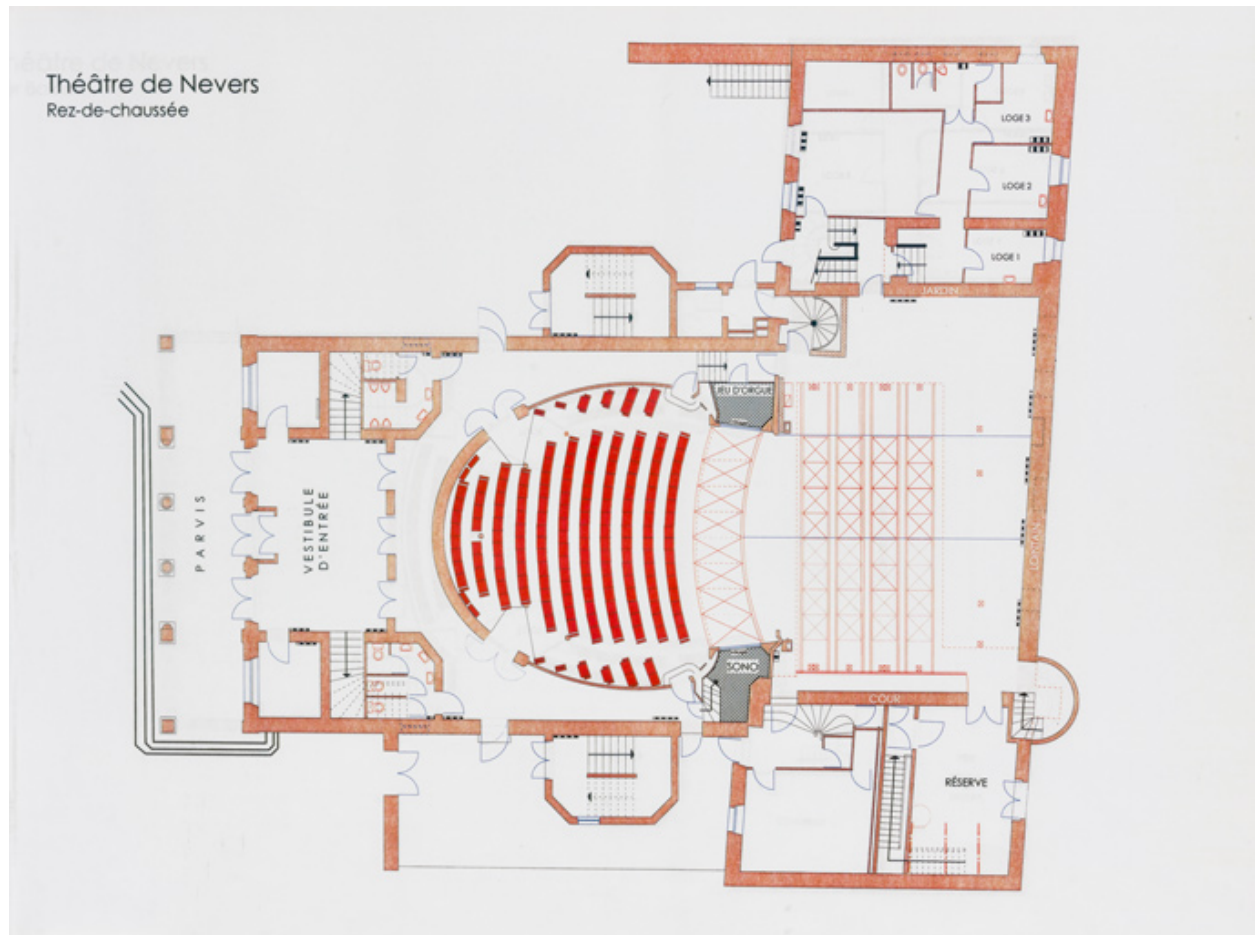
Théâtre de Nevers. Etat des lieux. Rez-de-chaussée. S.d. [octobre 2005].
