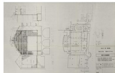
Ville de Nevers. Théâtre municipal. Mise en conformité. 1A. Plan des dessous de scène. Coupe transversale sur baie scène. Coupe longitudinale partielle. 1976. Phot. Pierre-Marie Barbe-Richaud, Autr. Camille Demangeat, Autr. Michel Rioualec IVR26_20245800467NUC4A
