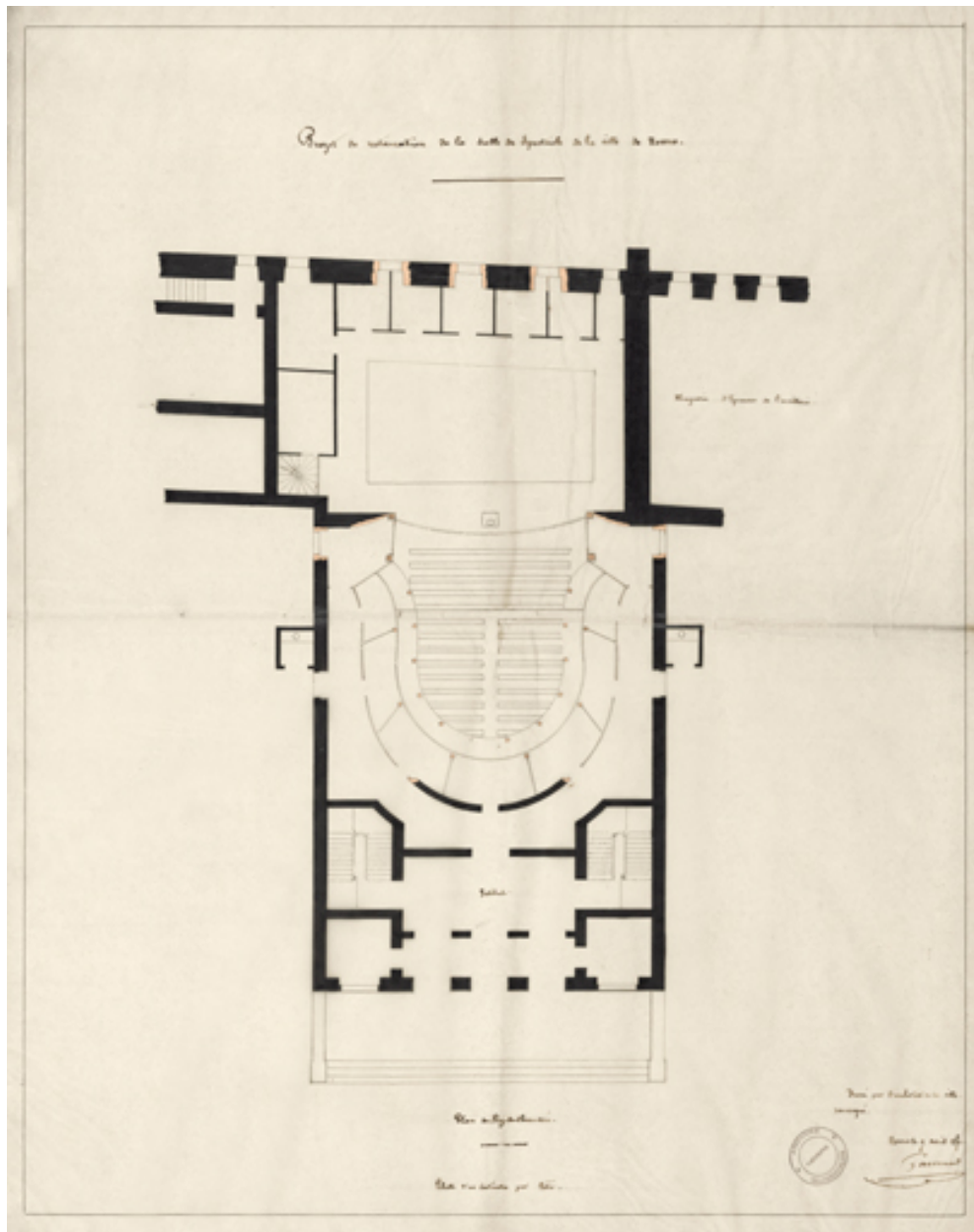
Projet de restauration de la salle de spectacle de la ville de Nevers. Plan du rez-de-chaussée. 9 avril 1851.
