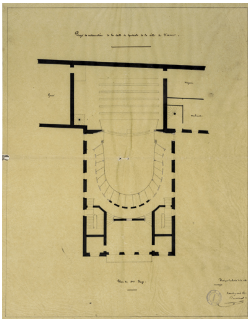
Projet de restauration de la salle de spectacle de la ville de Nevers. Plan du 2ème étage. 9 avril 1851.
