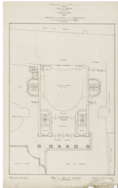
Théâtre. Projet d'escaliers de dégagement et de terrasse en avant de la façade. Plan du Rez-de-chaussée. [Mai-juin] 1897. Phot. Pierre-Marie Barbe-Richaud, Autr. Charles Brazeau IVR26_20245800432NUC4A
