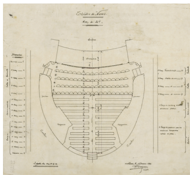
Théâtre de Nevers [implantation des loges et des sièges]. Rez-de-ch[auss]ée. 18 janvier 1899. Phot. Pierre-Marie Barbe-Richaud, Autr. Charles Brazeau IVR26_20245800438NUC2A
