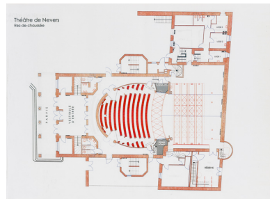
Théâtre de Nevers. Etat des lieux. Rez-de-chaussée. S.d. [octobre 2005]. Phot. Pierre-Marie Barbe-Richaud, Autr. auteur inconnu IVR26_20245800472NUC4A
