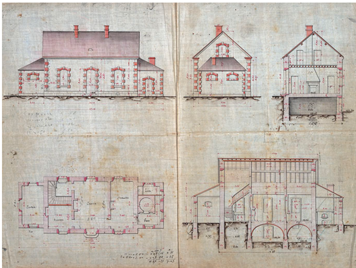
Achèvement du bief d'Apremont - Maison du barragiste (1882).
