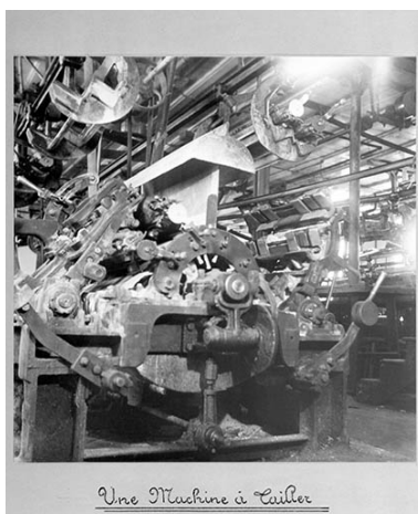
Une machine à tailler. Phot. Jérôme Mongreville IVR43_19923900025X
