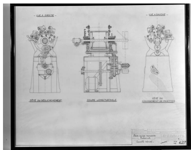
Petite équipe [à] marcassite. Machine à polir. Ensemble définitif, coupe et élévations. Phot. Jérôme Mongreville, Autr. René Chambard IVR43_19923900155V
