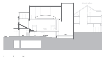
Coupe longitudinale. D'après une coupe fournie par la Communauté de l'Auxerrois, Patrimoine et aménagement de l'espace public. Dess. Aline Thomas IVR26_20248900081NUDA
