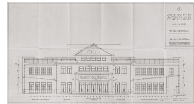
1. Salle des fêtes et patronages rue Joubert. Façade principale. 5 avril 1937. Phot. Pierre-Marie Barbe-Richaud, Autr. Georges Simonot IVR26_20238900778NUC2A
