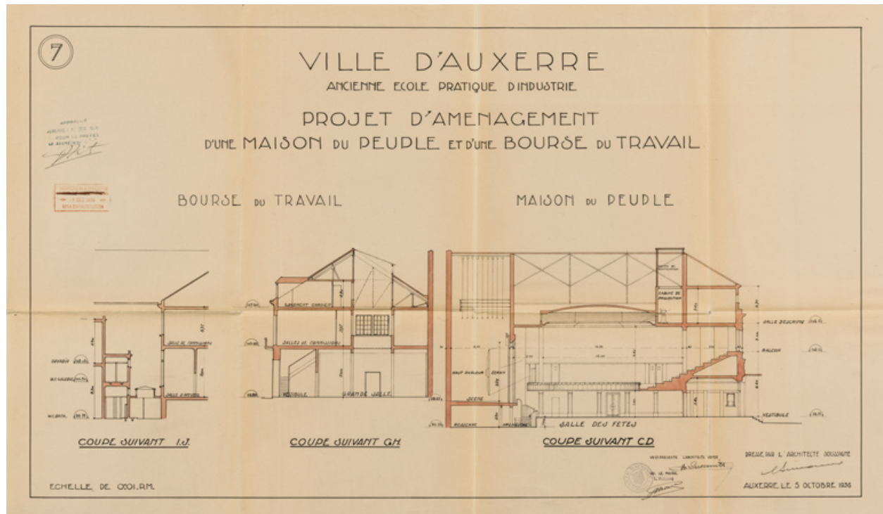
Projet d'aménagement d'une maison du peuple et d'une bourse du travail. 7. Bourse du travail [et] Maison du peuple [coupes]. 5 octobre 1936.
