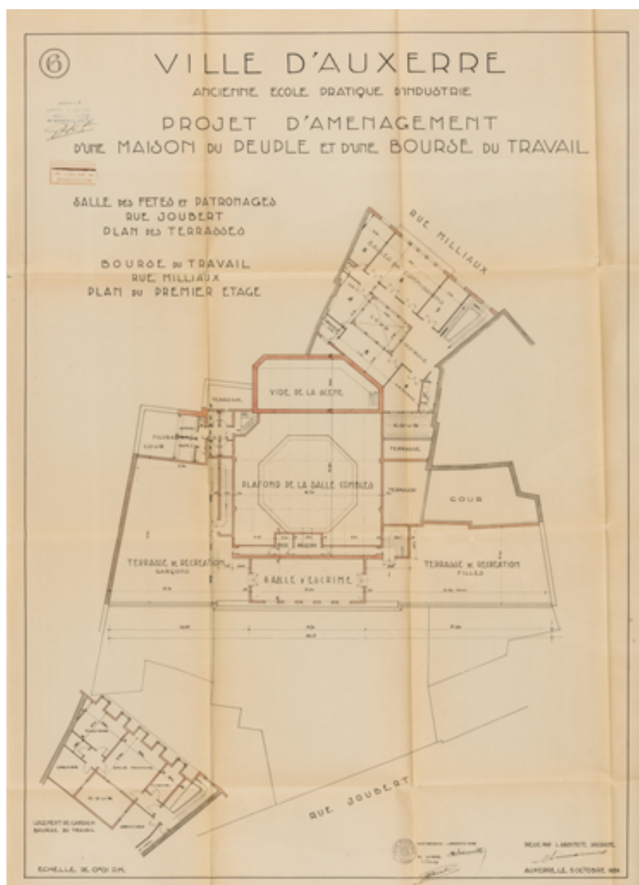
Projet d'aménagement d'une maison du peuple et d'une bourse du travail. 6. Salle des fêtes et patronages rue Joubert, plan des terrasses. Bourse du travail rue Milliaux, plan du premier étage. 5 octobre 1936.
