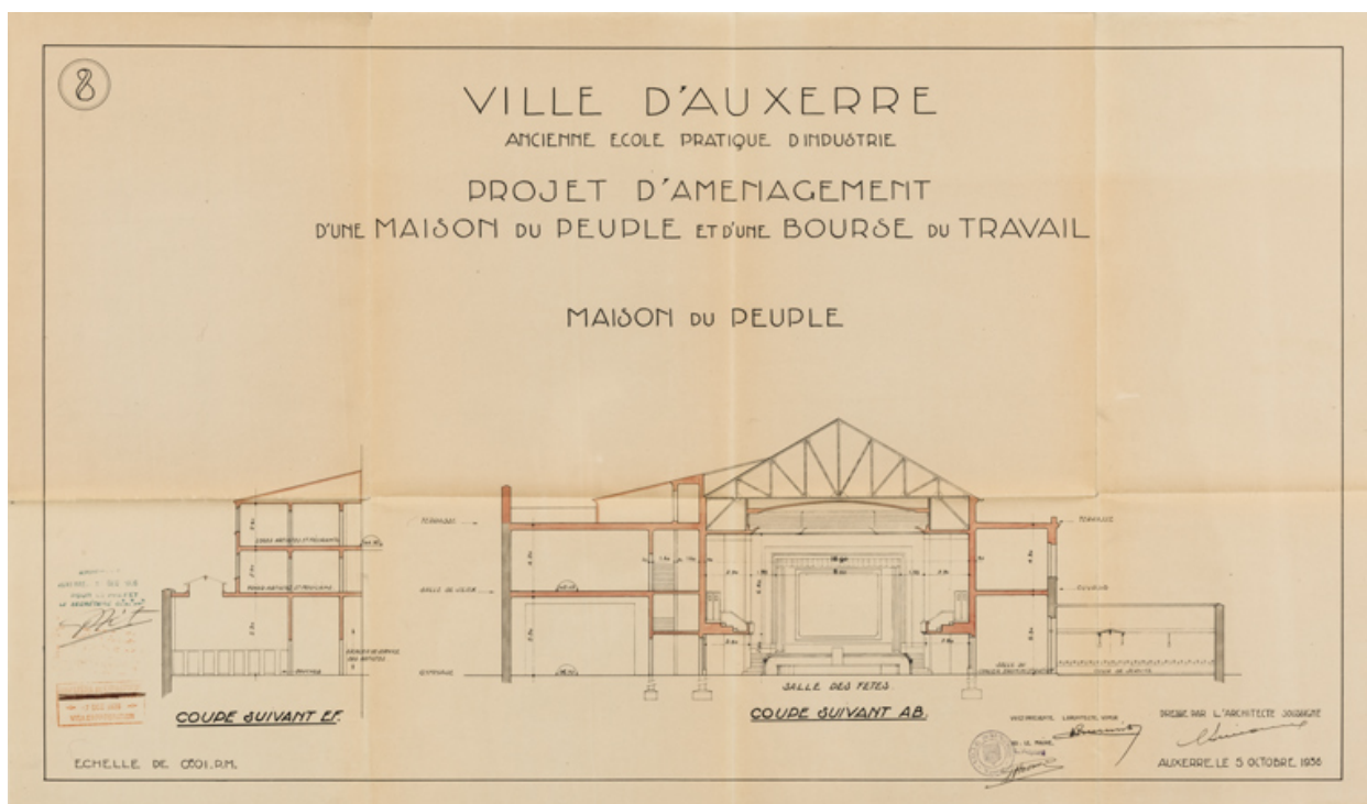
Projet d'aménagement d'une maison du peuple et d'une bourse du travail. 8. Maison du peuple [coupes]. 5 octobre 1936.
