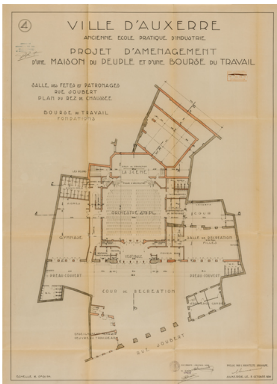
Projet d'aménagement d'une maison du peuple et d'une bourse du travail. 4. Salle des fêtes et patronages rue Joubert, plan du rez-de-chaussée. Bourse du travail rue Milliaux, fondations. 5 octobre 1936.
