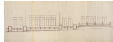
Ville d'Auxerre. Théâtre municipal. Projet de grille. 15 décembre 1952. Phot. Pierre-Marie Barbe-Richaud, Autr. Georges Simonot IVR26_20238900791NUC2A
