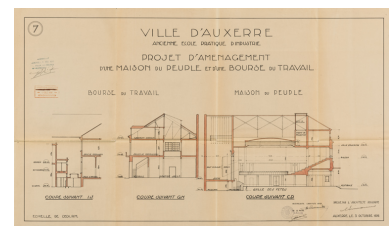
Projet d'aménagement d'une maison du peuple et d'une bourse du travail. 7. Bourse du travail [et] Maison du peuple [coupes]. 5 octobre 1936. Phot. Pierre-Marie Barbe-Richaud, Autr. Georges Simonot IVR26_20238900810NUC4A
