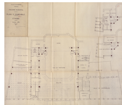
Ville d'Auxerre. Théâtre municipal [plans]. Etages. S.d. [1952 ?]. Phot. Pierre-Marie Barbe-Richaud, Autr. Georges Simonot IVR26_20238900784NUC2A
