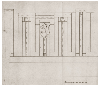
[Mur de clôture et de sa grille. Détail]. S.d. [1939]. Phot. Pierre-Marie Barbe-Richaud, Autr. Georges Simonot IVR26_20238900806NUC2A
