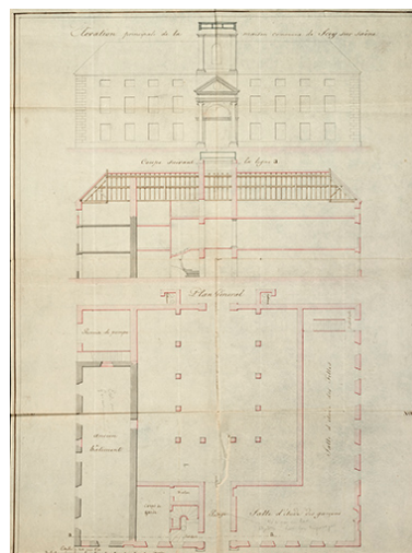
Élévation principale de la maison commune de Scey- sur-Saône. Coupe. Plan général [du rez-de-chaussée]. [1831]. Autr. Pierre Duret, Repro. Jérôme Mongreville IVR43_20197000003NUC4A
