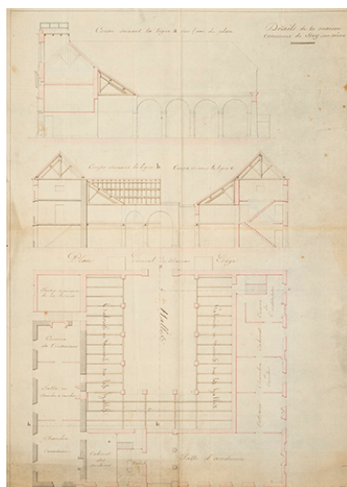
Détails de la maison commune de Scey-sur-Saône. Coupe. Plan général du premier étage. [1831]. Autr. Pierre Duret, Repro. Jérôme Mongreville IVR43_20197000005NUC4A
