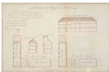
Projet des travaux à faire pour la construction d'une maison destinée à l'établissement de l'école des filles et pour la reconstruction des halles. [Plans du rez-de-chaussée et de l'étage, coupes]. [1831]. Repro. Jérôme Mongreville, Autr. Pierre Duret IVR43_20197000004NUC4A
